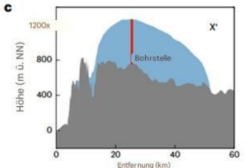
c, Querschnitt zeigt Eisdicke und Felsuntergrundtopographie des Prudhoe Dome
