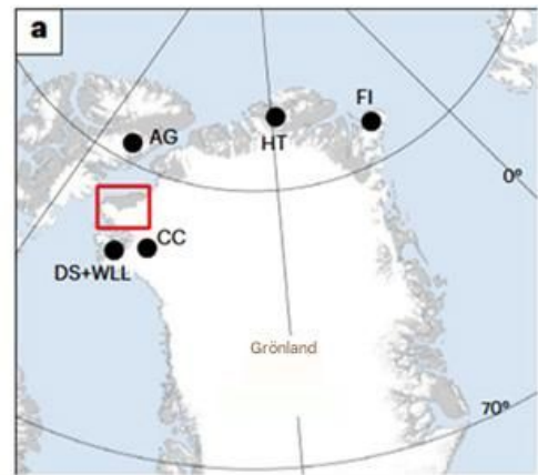
Abb. 1a Nord des Untersuchungsgebiets. a, Karte von Grönland und Umgebung mit den heutigen Ortsbezeichnungen. Das Untersuchungsgebiet ist rot umrandet, und die Standorte der Eiskappen Hans-Tausen (HT) und Flade-Isblink (FI, der Eiskappen-Standard-Camp-Century (CC), der Eiskappen-Standard-Agassiz-Eiskappe (AG) sowie der Seen Deltase (DS) und Wax Lips (WLL) sind eingezeichnet.
