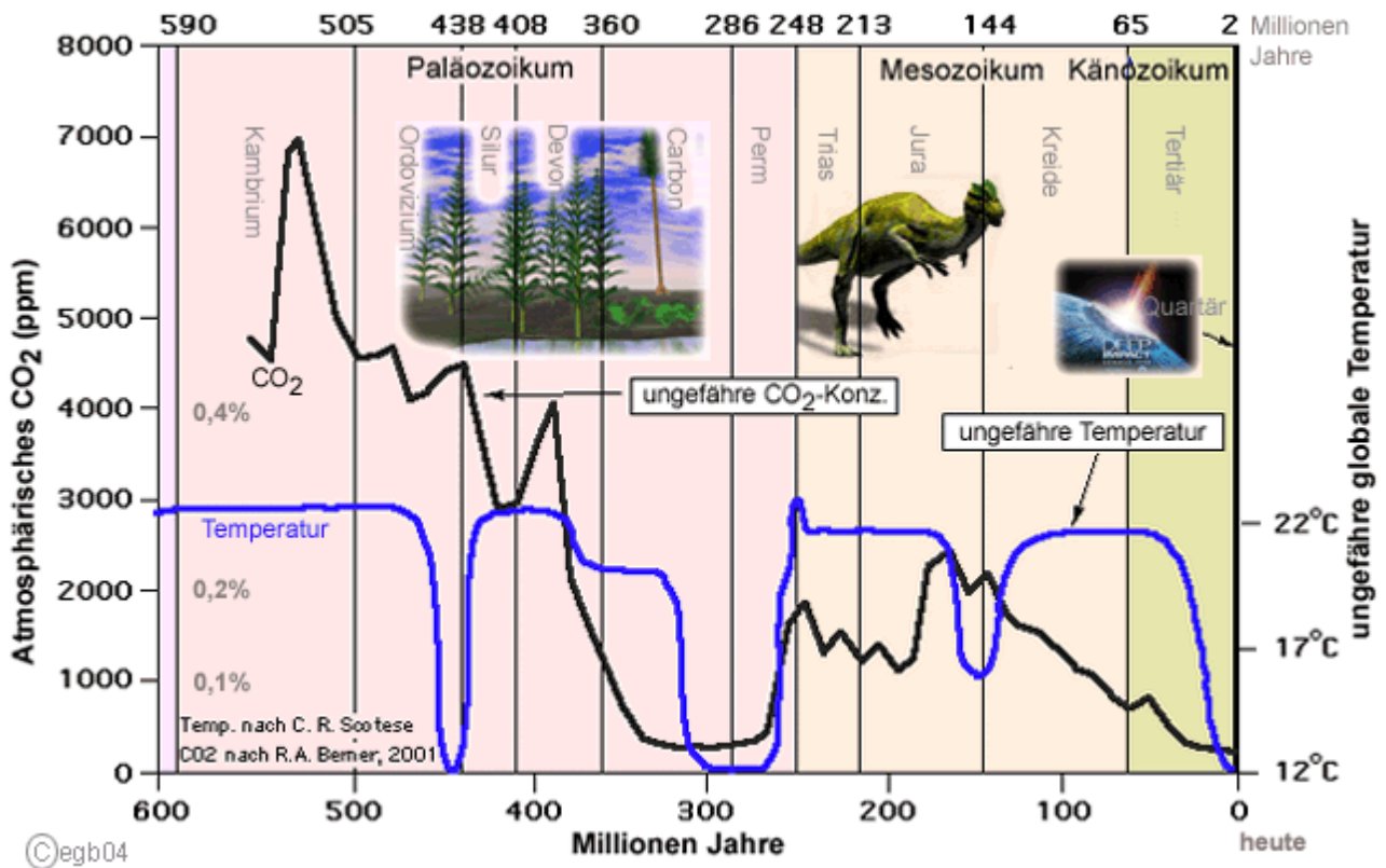
Bild 1: Zeitliche Entwicklung der CO 2 -Gehalte in der Atmosphäre sowie der Temperaturen
