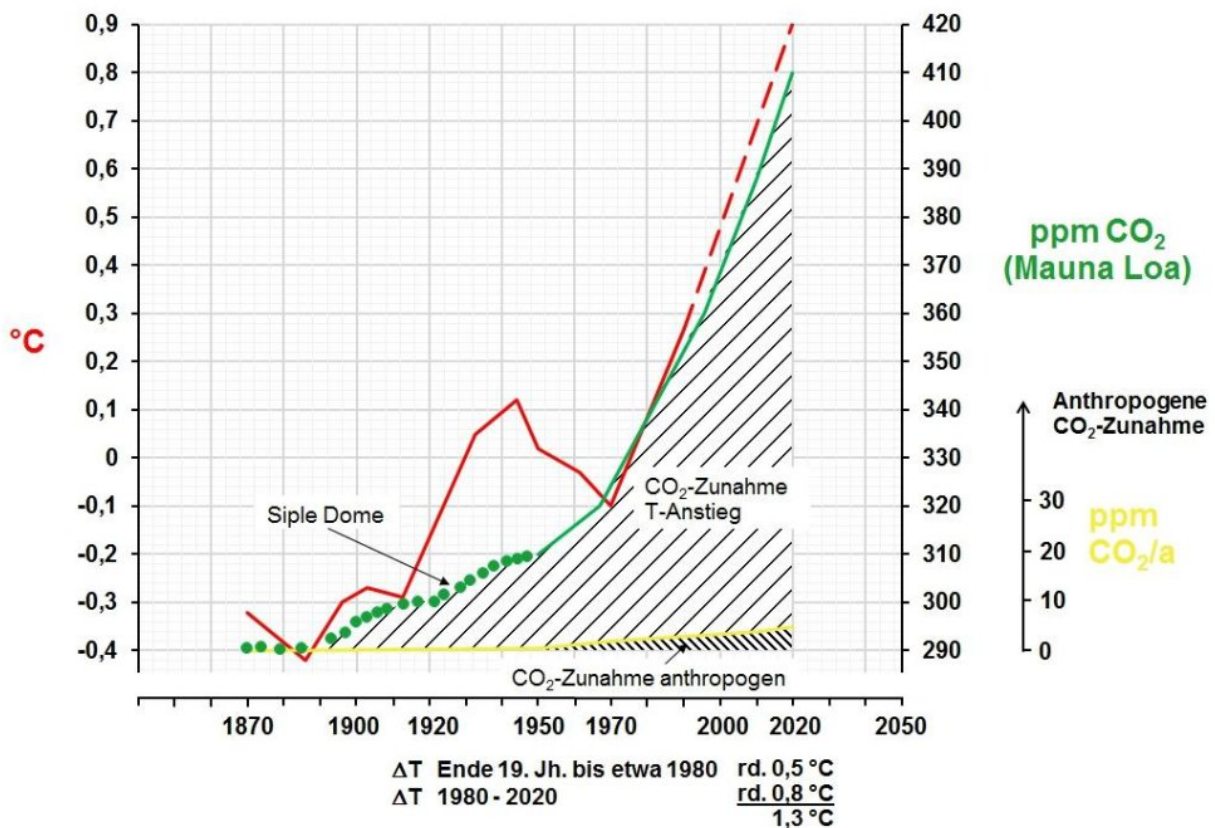
Bild 7: Entwicklung der Gesamt-CO 2 -Konzentrationen der Atmosphäre sowie der über die anthropogenen CO 2 -Emissionen errechnete CO 2 -Anteil
