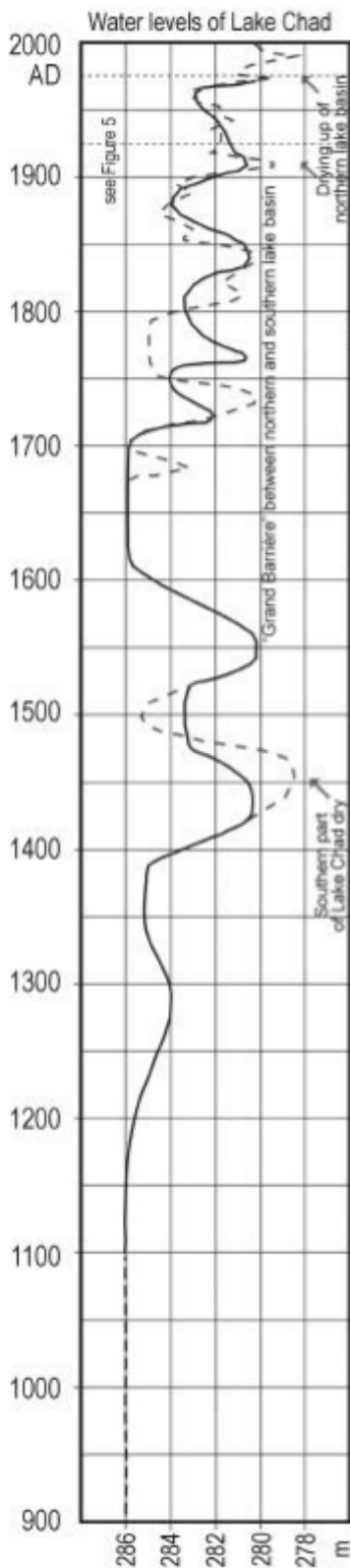
Bild 21 [27] Verlaufsrekonstruktion des Pegels Tschad-See seit 900
