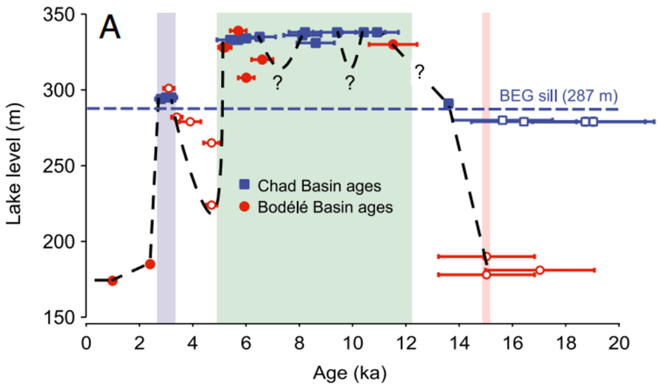
Bild 20 [28] Fig. 2 The lake-level history of Lake Mega-Chad. Verlaufsrekonstruktion des Pegels Tschad-See seit 16tausend Jahren
