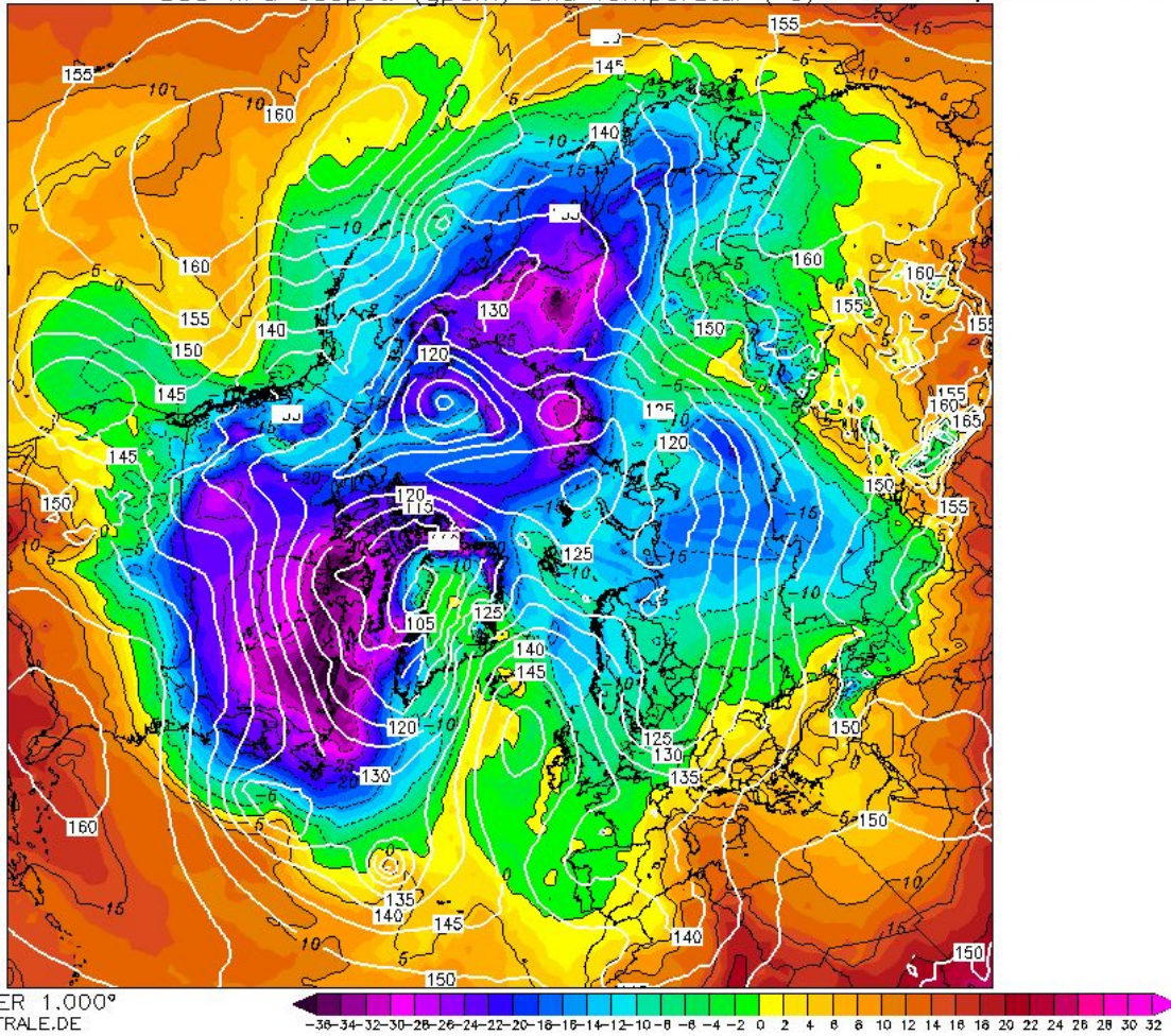
Abbildung 2: Temperatur im 850-hPa-Niveau vom 25. Februar 2023, 00 UTC. Der Kältepol über Kanada sticht deutlich hervor (im linken Teil des Bildes). Quelle: Wetterzentrale.de
