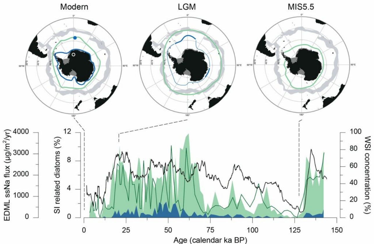
Abbildung 4. Unten: Natriumgehalt in Eiskernen (schwarze Linie) und Diatomeendaten, die die vergangenen Winter- (grün) und Sommerbedingungen (blau) des Meereises zeigen. Oben: Karten der durchschnittlichen Winter- (grün) und Sommergrenzen (blau) des Meereises für heute, das letzte glaziale Maximum (~20.000 Jahre vor heute) und die warme letzte Zwischeneiszeit (~125.000 Jahre vor heute). Die graue Zone markiert die moderne Polarfront. Die Kernstandorte sind auf der modernen Karte dargestellt (blauer Punkt = Meereskern, weißer Kreis = Eiskern).
