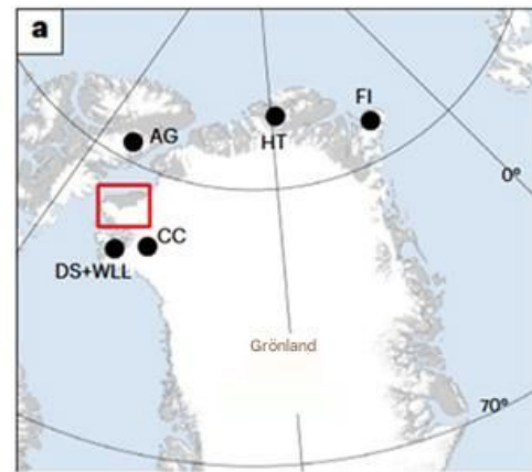
Abb. 4 Karten des Untersuchungsgebiets. a, Karte von Grönland und Umgebung mit den heutigen Staatsgrenzen. Das Untersuchungsgebiet ist rot umrandet, und die Standorte der Eiskappen Hans-Tausen (HT) und Foulke-Eiskappe (FI), der Eiskappen-Standard-Century (CC), der Eiskappen-Standard-Agassiz-Eiskappe (AG) sowie der Seen Deltase (DS) und Wax Lips (WLL) sind eingezeichnet.
