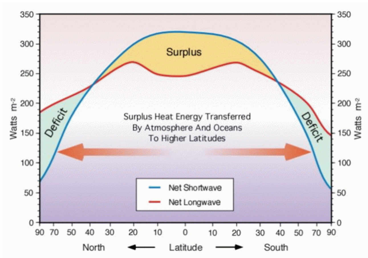
Abbildung 3: Durchschnittliche Wärmeüberschüsse/-defizite über ein Jahr auf der Erde und der damit verbundene advective Wärmetransport, den ein stabiles Klima erfordert. [7]
