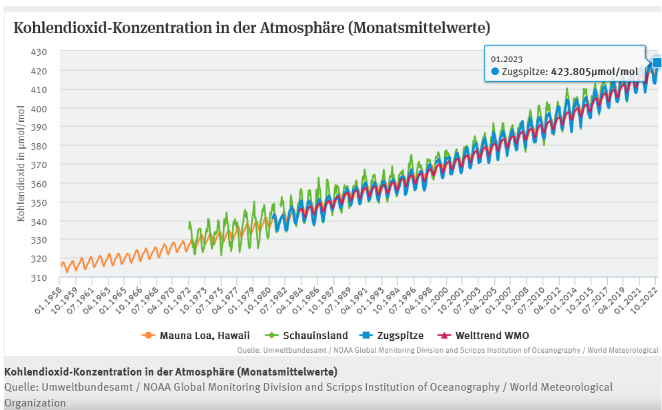
Abb.3: Die CO 2 -Konzentration der Atmosphäre steigt stetig an. Ganz im
