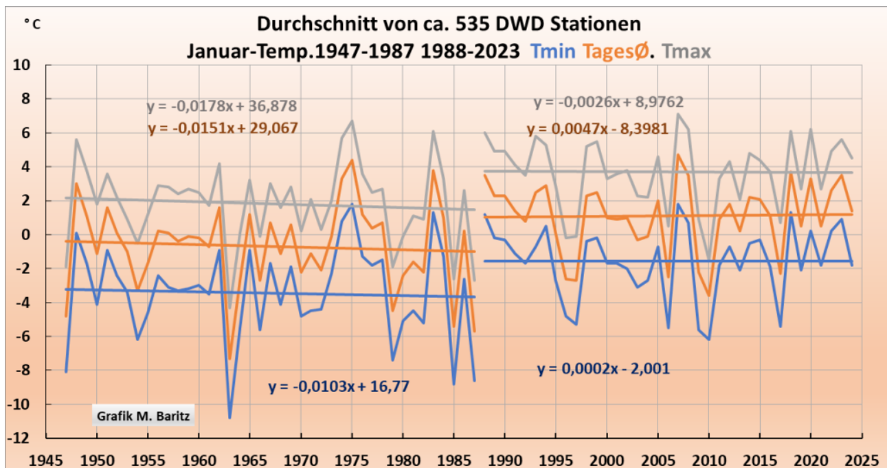
Abb.2: Die mittleren braunen Grafiklinien entsprechen dem Verlauf von Abb.1. Die Formeln unterscheiden sich ganz leicht, weil hier nur 535 Stationen geführt werden. Es liegen nicht mehr vor, die zugleich auch T_{max} und T_{min} erfassen.
