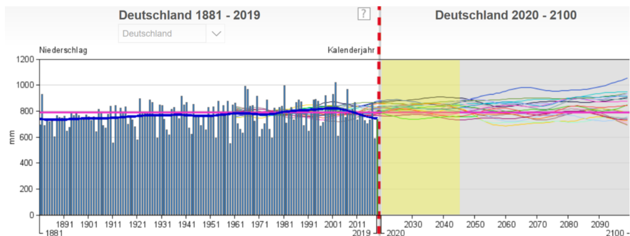
Bild 1 Screenshot vom DWD Klimaatlas. Niederschlag Deutschland mit Projektionsläufen von Klimasimulationen. Kein Simulationslauf trifft die
