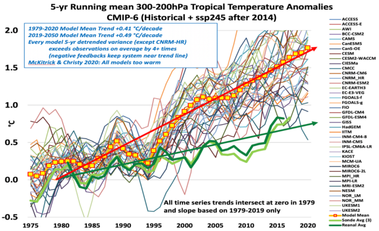
Bild 4 Ergebnisse von 32 Computermodellen des IPCC für Temperaturverläufe in den Tropen. Die dicke rote Kurve ist deren Mittelwert. Im Vergleich dazu wurden in der dicken grünen Kurve die realen, durch Ballonmessungen gewonnenen Daten eingetragen.
