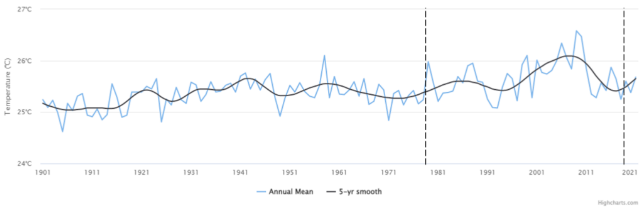
Bild 11 Temperaturverlauf Bangladesch. Vom Autor eingezeichnet der Zeitraum der Beobachtungsdaten. Quelle: World Bank Group Climate Change Knowledge Portal
