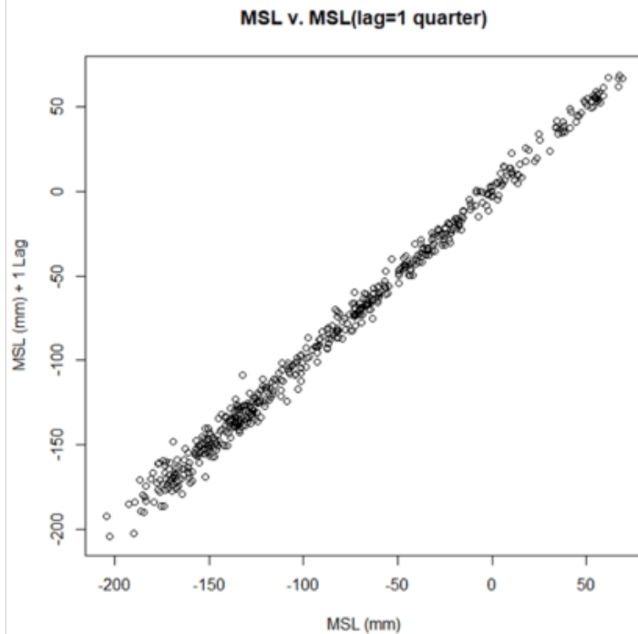
Abbildung 2. Aufzeichnung der GMSL gegen die vorherige GMSL, die erste Verzögerung. Die Werte sind stark korreliert. Die kleine Autokorrelationskurve zeigt, dass die GMSL seit mindestens 7 Jahren stark autokorreliert ist.
