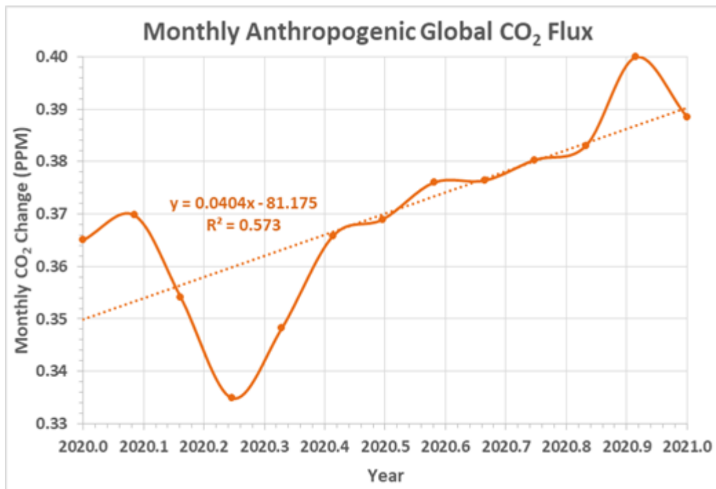
Abbildung 1: Monatlicher anthropogener CO 2 -Eintrag mit Trendlinie
