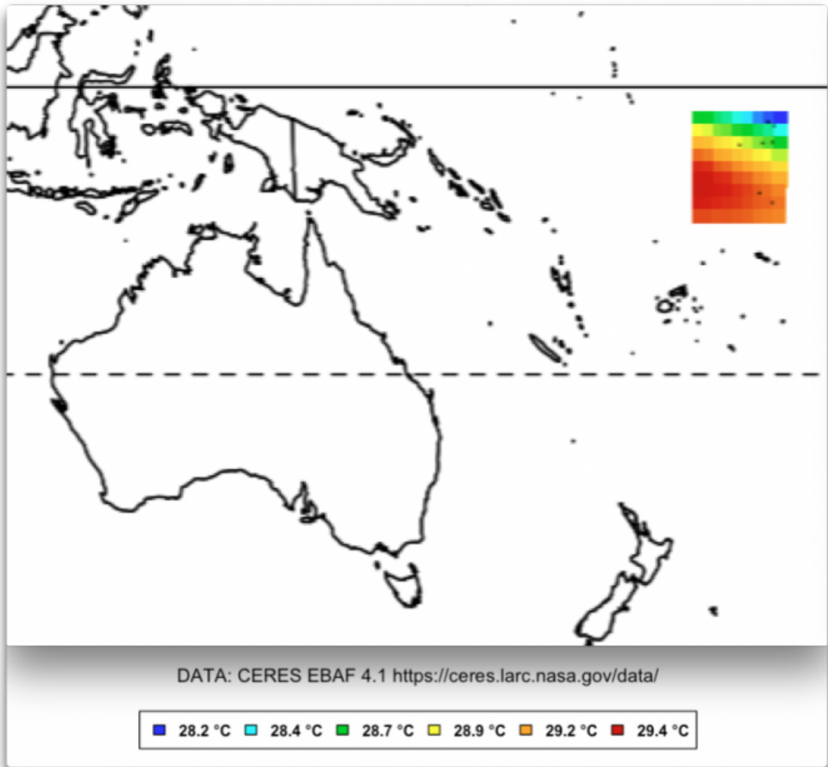
Abbildung 3a: Temperatur eines 9°-Gitterquadrats im Pazifik.
