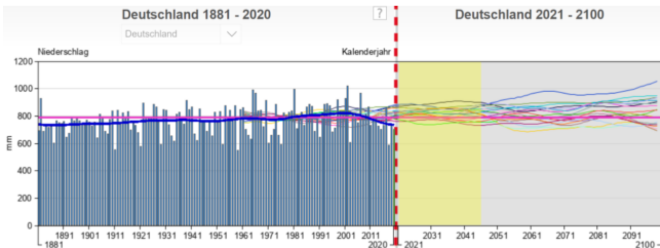
Bild 9 Deutschland, Jahresniederschlag von 1881 – 2100. Quelle: DWD-Datenviewer
