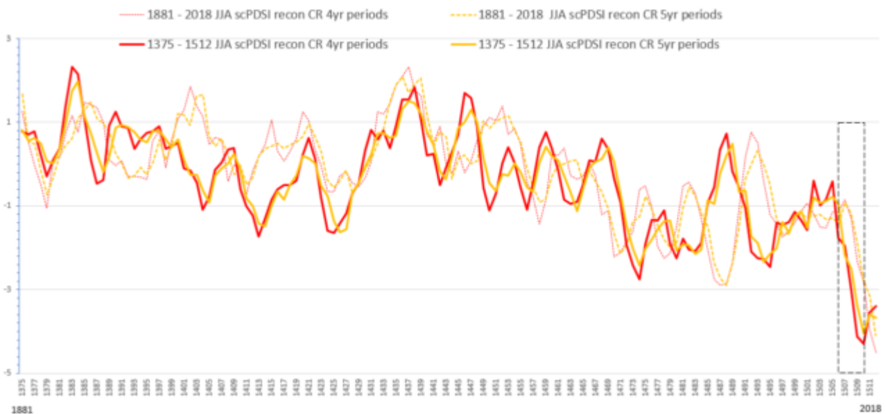
Bild 6 Sommervariabilität des Trockenheitsindexes von -1375 – 1512 und 1881 – 2018. Grafik vom Autor anhand der Daten [1] erstellt
