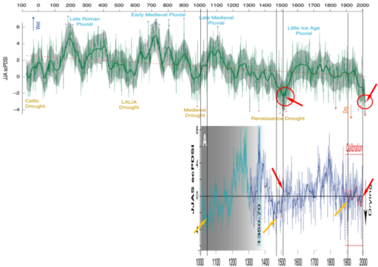
Bild 10 Zusammenstellung Büntgen 2020 [1] und Büntgen 2010 [4] im gleichen Maßstab. Grafik vom Autor erstellt
