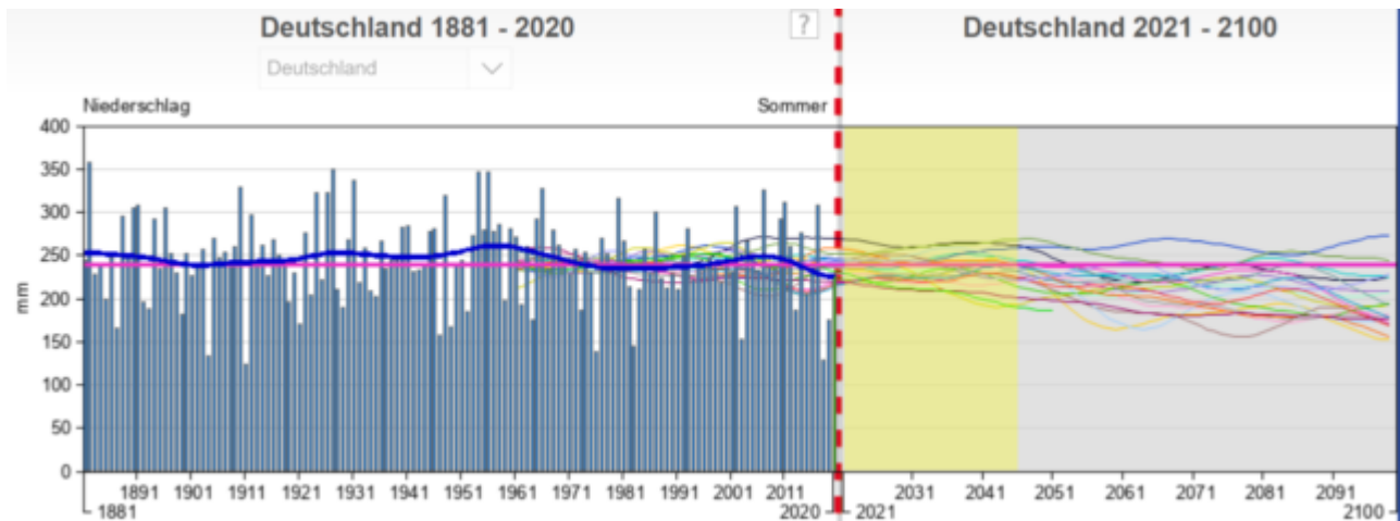
Bild 8 Deutschland, Sommerniederschlag von 1881 – 2100. Quelle: DWD-Datenviewer
