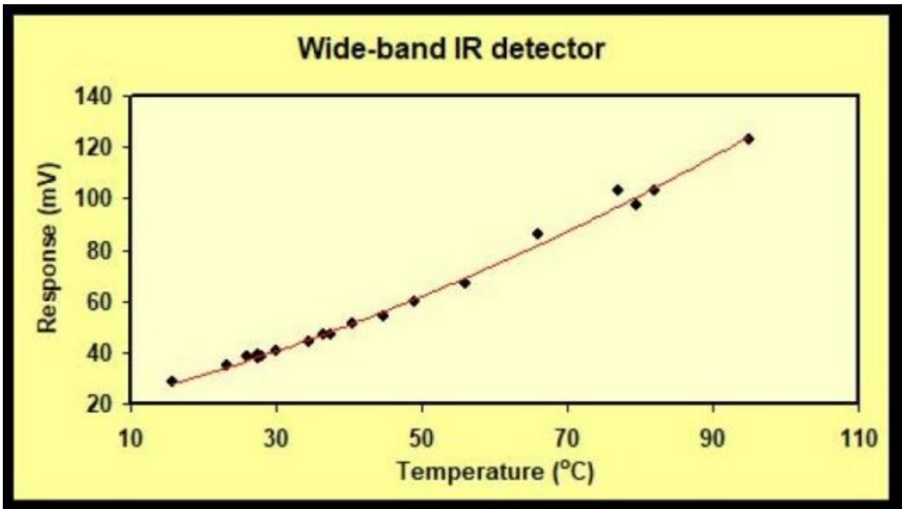
Abbildung 2: Temperatur-Kalibrierung
