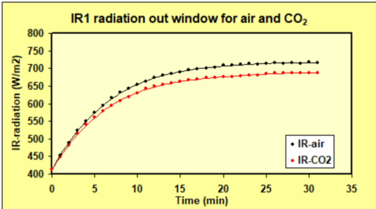
Abbildung 6: Absorption von IR-Strahlung. Bereich: 2,5 – 20 \mu\text{m} . Die Heizung erfolgt mit der Al-Platte.
