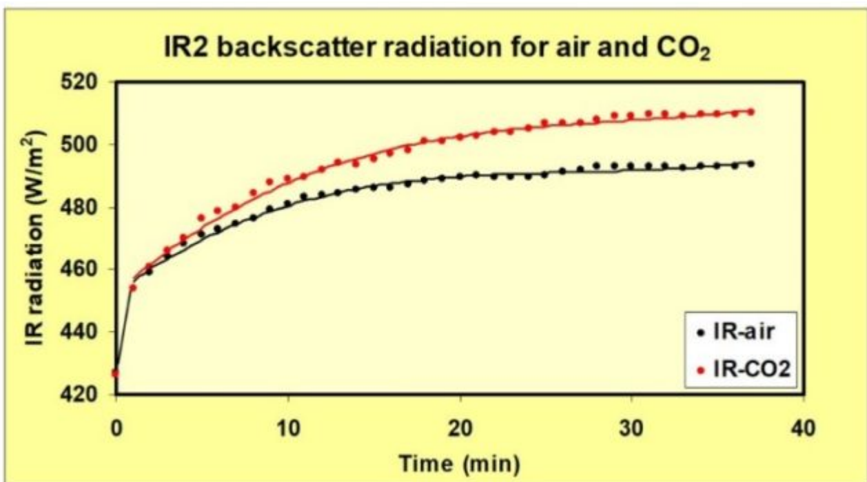
Abbildung 8: Die Rückstreuung (erhöhte IR-Strahlung, gemessen mit IR2), die von der Rückwand der Box empfangen wird, stieg um 17 W/m 2 mit CO 2 in der vorderen Box. Die Erwärmung erfolgt über die Al-Folie.
