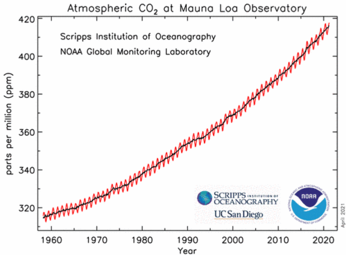
Grafik 3: Die Keeling-Kurve mit den Messwerten des atmosphärischen Gehalts an Kohlenstoffdioxid in der Atmosphäre, gemessen am Mauna Loa. Quelle Wikipedia
