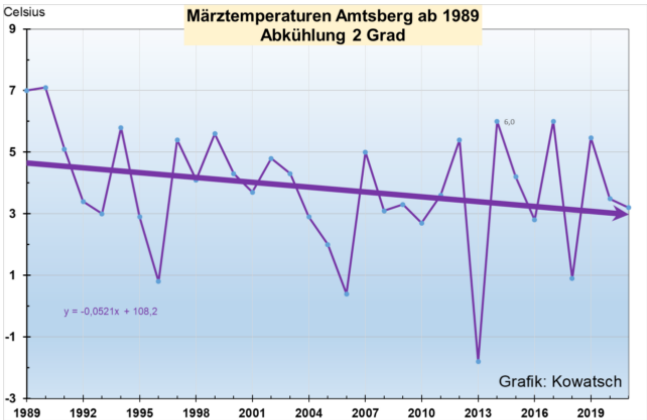
Abbildung 6: Bei der wärmeinselarmen Station Amtsberg wird der Monat März seit über 33 Jahren deutlich kälter und das trotz deutlicher Zunahme der CO 2 -Konzentrationen der Atmosphäre. Die fallende Trendlinie ist das Gegenteil einer behaupteten CO 2 -Erwärmung.
