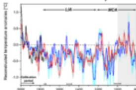
Temperaturrekonstruktionen aus der Studie
