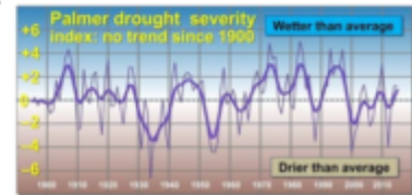
Grafik: Trockenheitsindex seit 1900 [136] Waldbrände 4 (19) - Klimafolgen-Berichterstattungen
