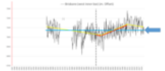
Pegeldaten Brisbane (Australien Ostküste) ab ca. 1965. Pegel auf das Jahr 2018 normiert. Datenquelle: PSMSL. Grafik vom Autor erstellt
