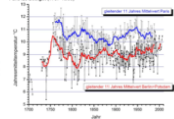
Vergleich Temperaturverlauf Berlin und Paris 1702 – 2007. Quelle: [1,2,3]
