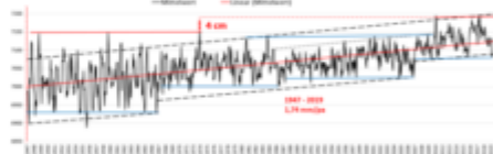
PSMSL-Datensätze: Mittelwert und Regressionsgeraden ab 1947. Pegel auf das Jahr 2018 normiert. Grafik vom Autor erstellt
