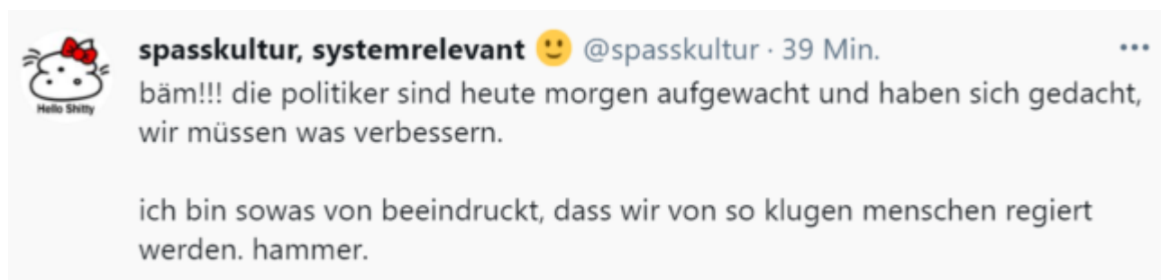
Bild 21 Tweet
