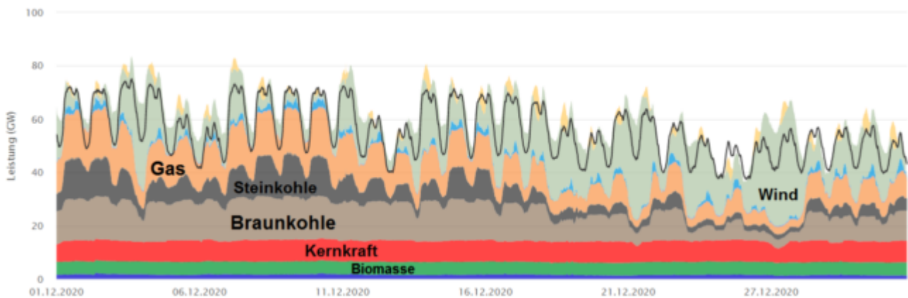
Nettostromerzeugung in Deutschland im Dezember 2020
