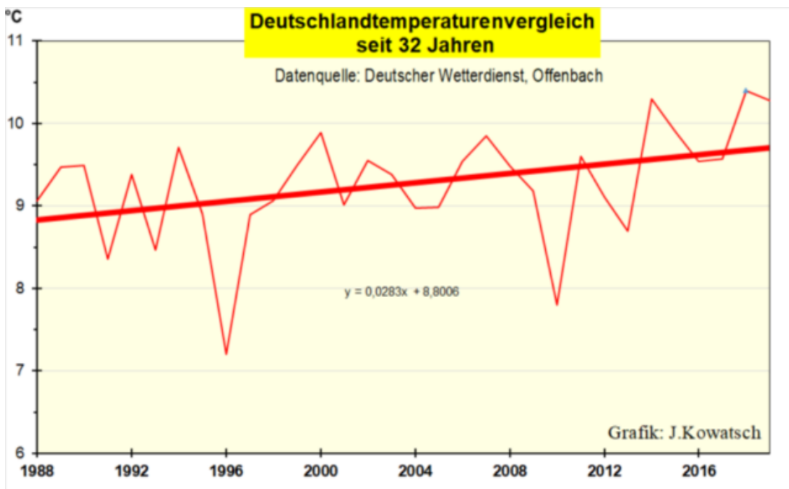
Abbildung 2: 1988 erfolgte bei allen Wetterstationen Deutschlands ein Temperatursprung auf ein höheres Niveau. Die Jahre wurden plötzlich wärmer. Und innerhalb dieses Zeitraumes bis heute sind die Temperaturen im Schnitt aller DWD-Wetterstationen weiter angestiegen. Das Jahr 2020 wird diesen Erwärmungstrend bestätigen. Voraussichtlicher Schnitt 2020 10,4
