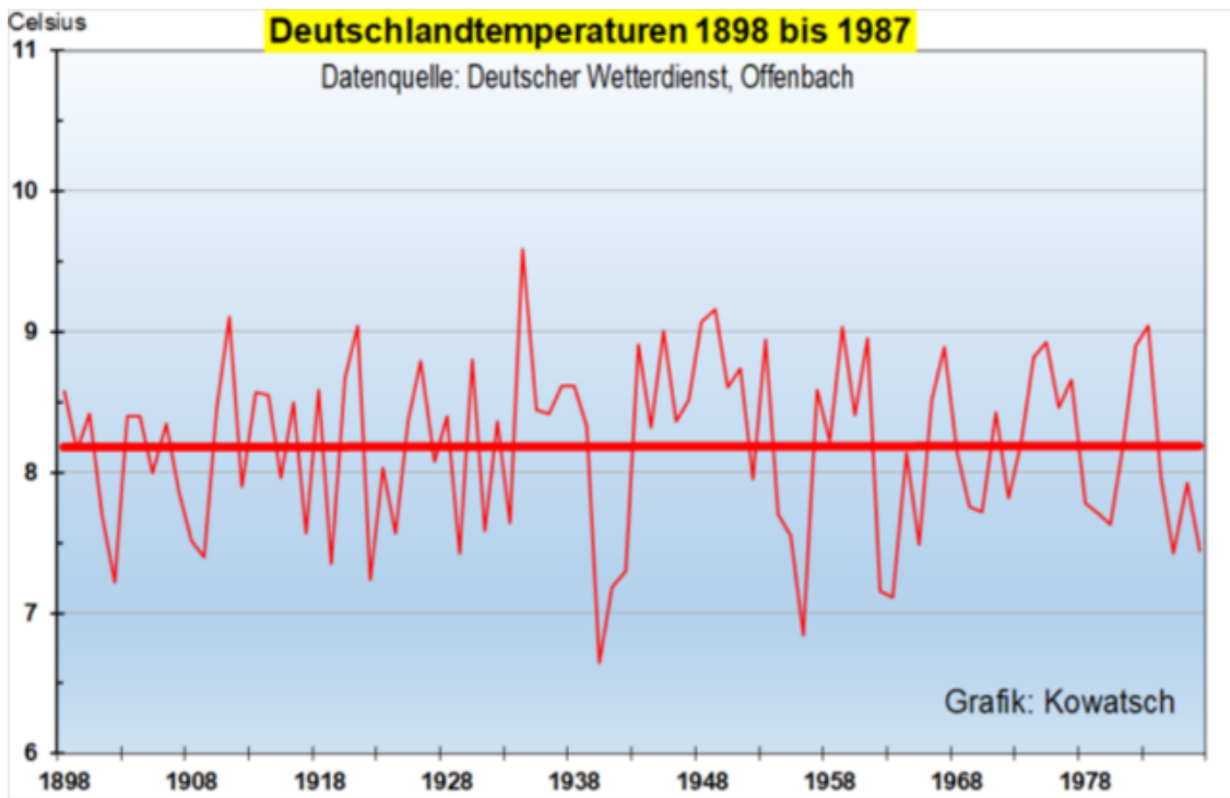
Abbildung 1 90 Jahre lang gab es laut DWD-Temperaturreihe keinerlei Erwärmung in Deutschland, trotz stark steigender CO 2 -Konzentrationen in der Atmosphäre. Hat die CO 2 -Erwärmungswirkung etwa 90 Jahre lang ausgesetzt?
