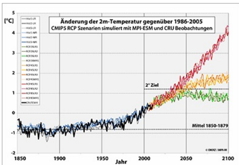
Abb.1 : Das 2°-Ziel [2]
