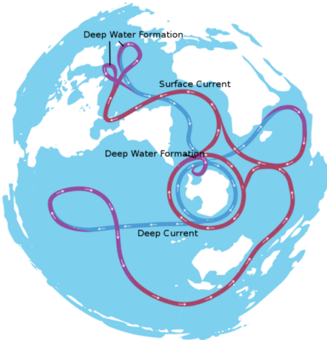
Abbildung 3. Die Hauptwege, die das Tiefenwasser auf seinem Weg von
