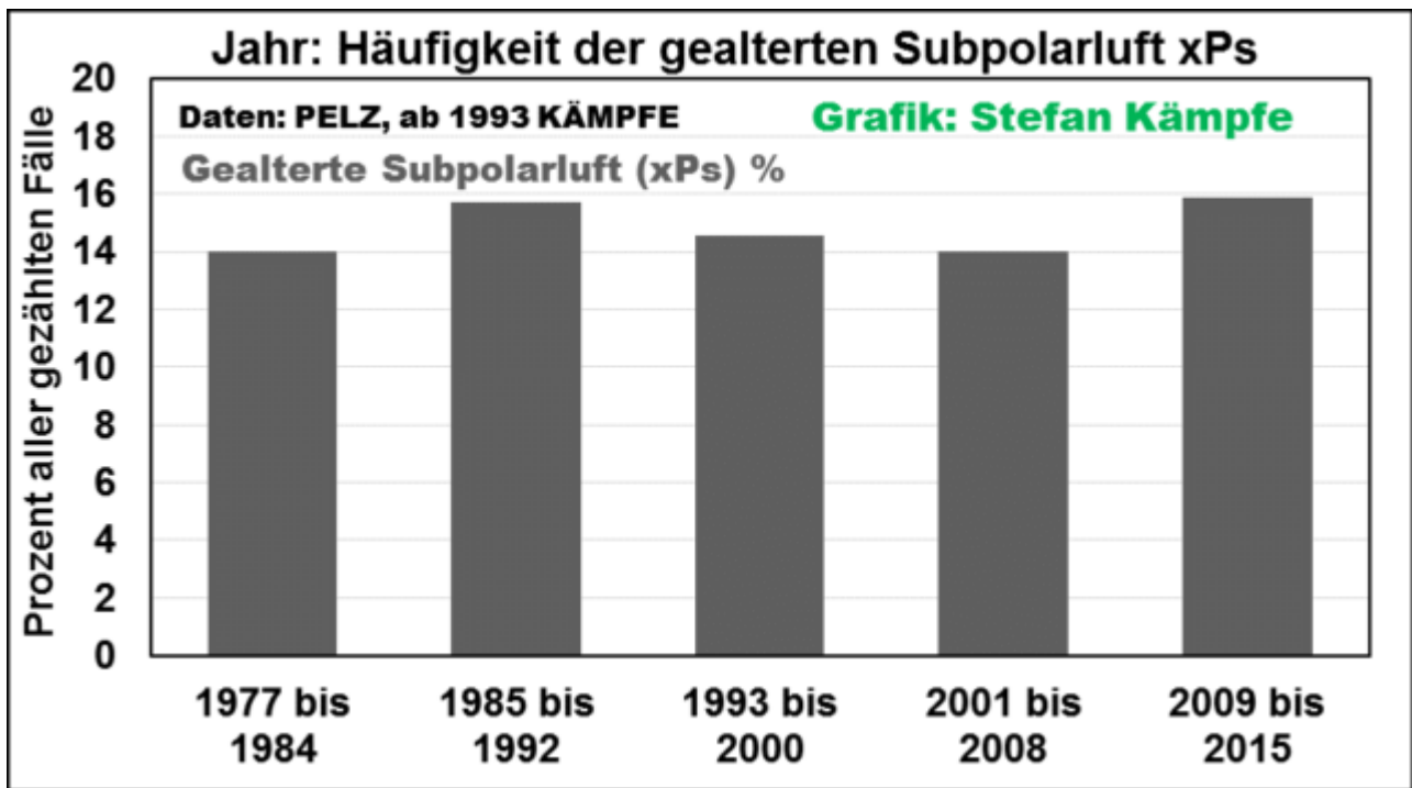
Abbildung 11: Die besonders nebelanfällige Luftmasse xPs wurde nicht seltener.
