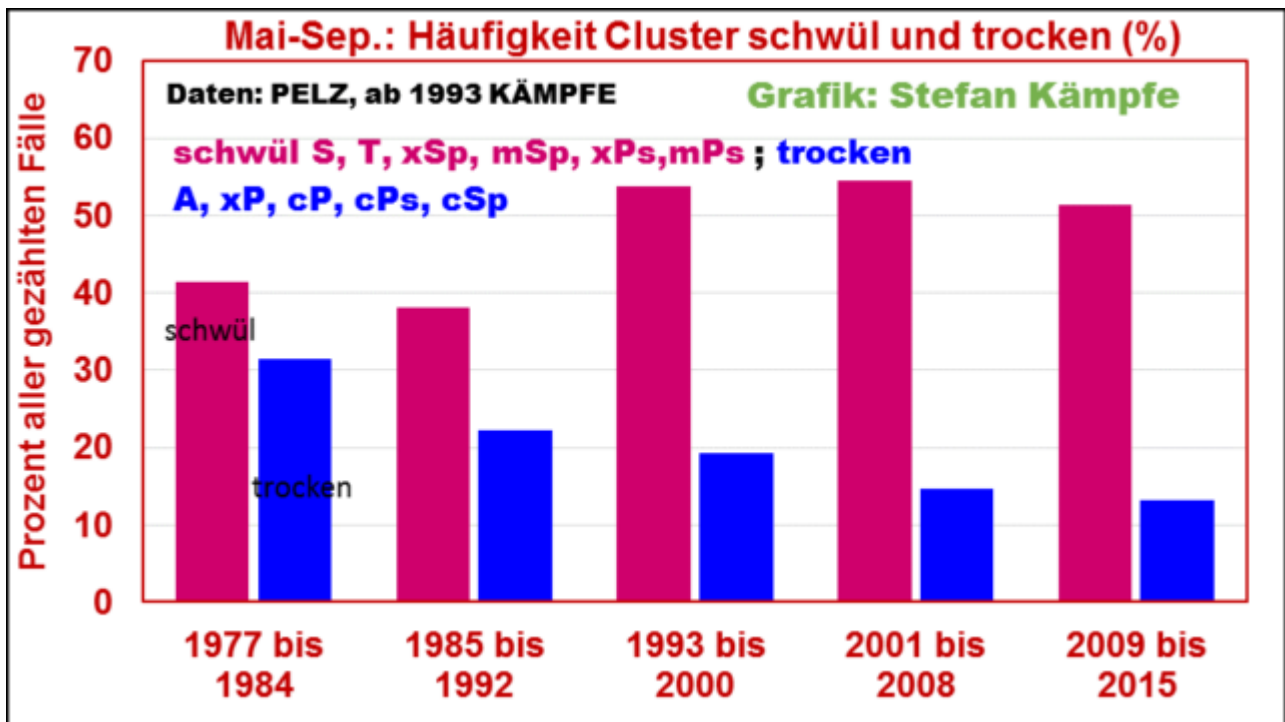
Abbildung 9: Auch hier zeigt sich der Klimasprung: Häufung schwüler und Abnahme wasserdampfer Luftmassen ab den 1990er Jahren; danach passierte aber nichts Dramatisches mehr.
