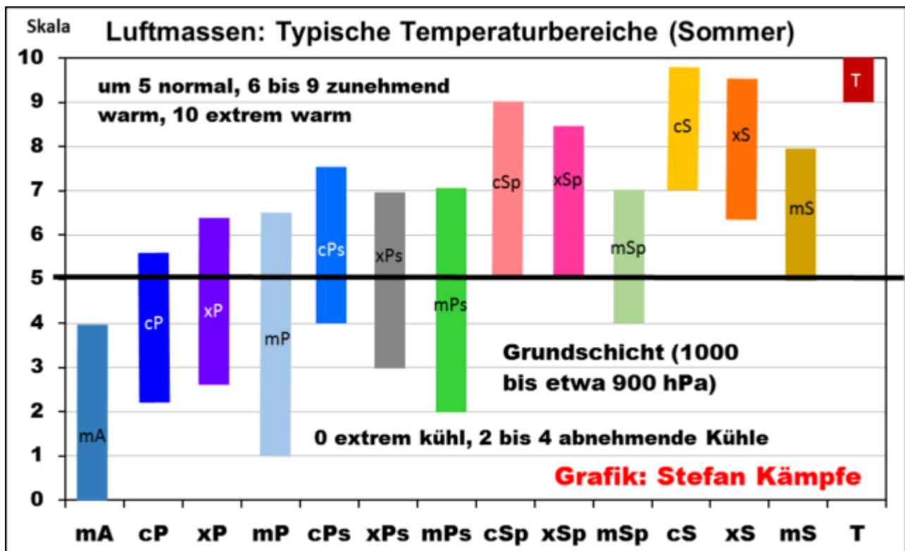
Abbildungen 7a und b: Temperaturintervalle der Luftmassen in den beiden Hauptjahreszeiten Winter (7a, oben) und Sommer (7b, unten) nach den Erfahrungen des Autors. Die großen Variationen resultieren im Winter vor
