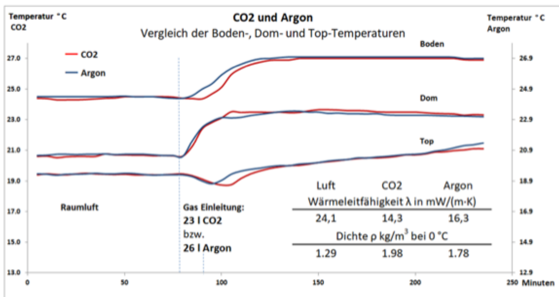
Abb. 4: Vergleich der \text{CO}_2 - und der Argon-Temperatur-Anstiege
