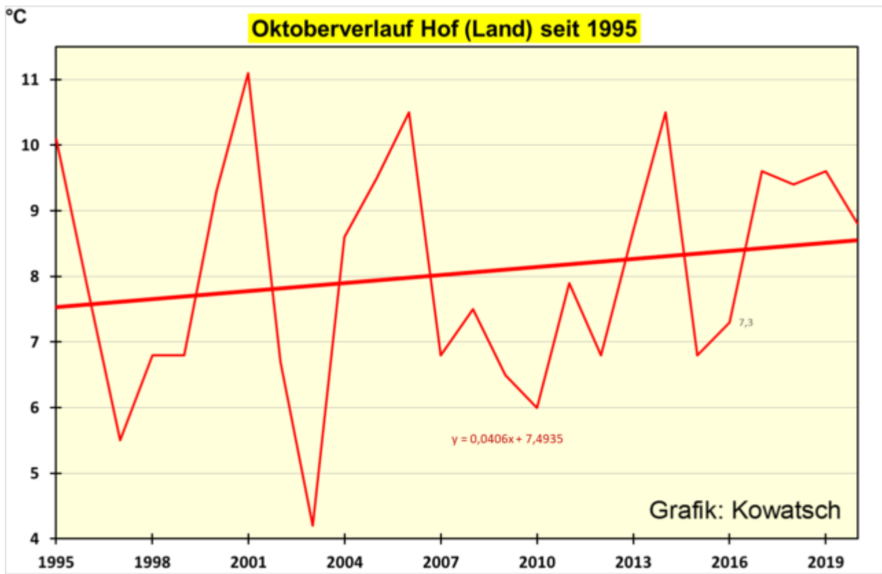
Abb. 6: Die Umgebung der Wetterstation Hof, einst ländlich und westlich der Stadt wurde nach der Wende mit einem Gewerbegebiet umbaut, deshalb hält die Erwärmung auch seit 1995 weiter an. Ein eindeutiger, vom Menschen verursachter und jährlich zunehmender WI-effekt. Das ist, wenn auch abgeschwächt, der Normalfall bei den meisten der 1900 Wetterstationen.
