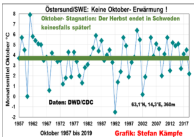
Abb. 11: In Östersund (westliches Mittelschweden am Ostfuß des Skandinavischen Gebirges) bleibt der Oktober ein empfindlich kühler Herbstmonat. Was würde wohl Greta sagen, wenn man ihr diese Grafik ihres Heimatlandes zeigen würde und zugleich die Grafik des CO 2 -Anstieges?
