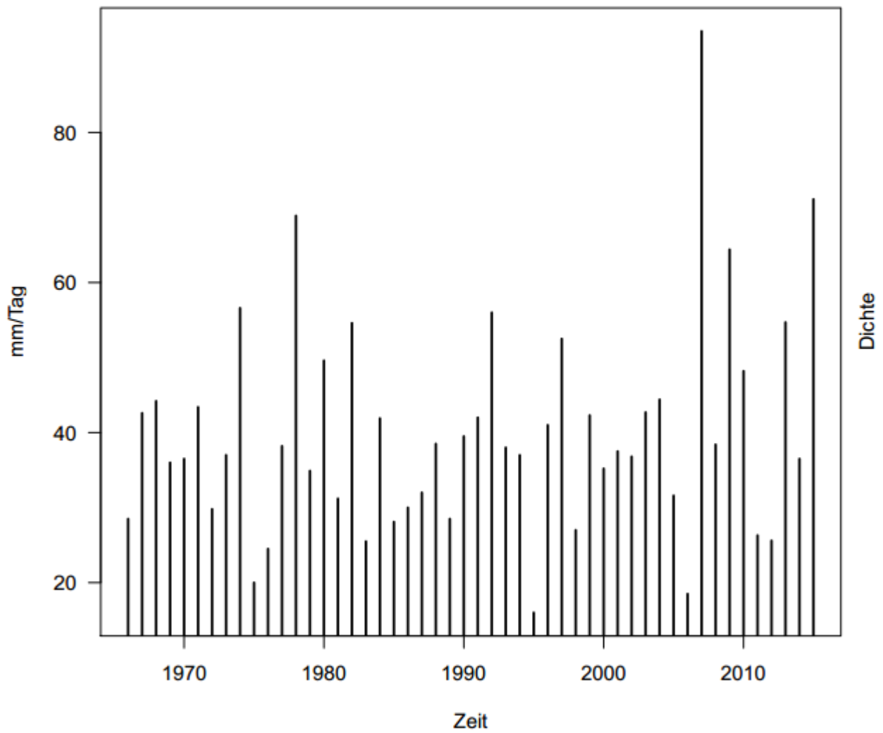
Bild 23 CH Aarberg, 1-Tages-Niederschlag 1966 – 2015
