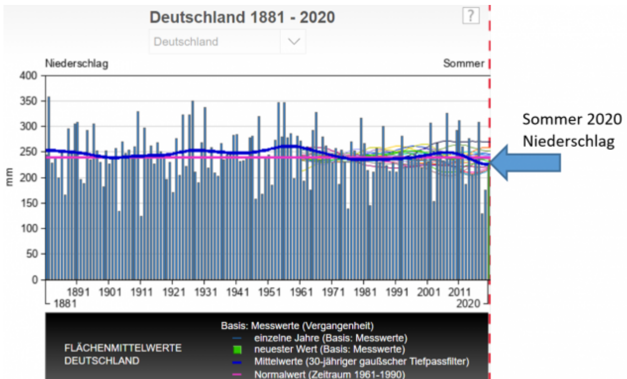
Bild 9 Deutschland, Sommer-Niederschlag 1881 – 2020. Quelle: DWD-Viewer
