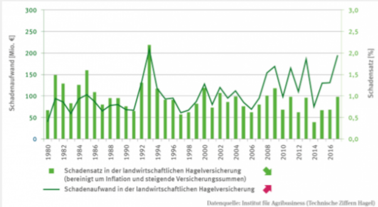
Bild 19 Deutschland Hagelschäden: „Die Ereignisse zeigen einen fallenden Trend“.Quelle: Deutscher Klima-Monitoringbericht 2019
