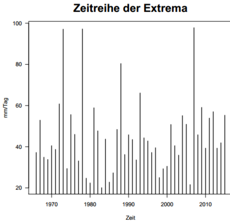
Bild 29 CH Zurich / Fluntern, 1-Tages-Niederschlag 1966 – 2015
