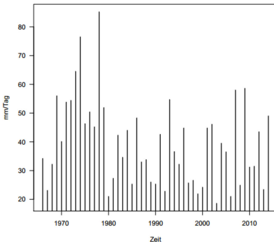
Bild 30 CH Weinfelden, 1-Tages-Niederschlag 1966 – 2015
