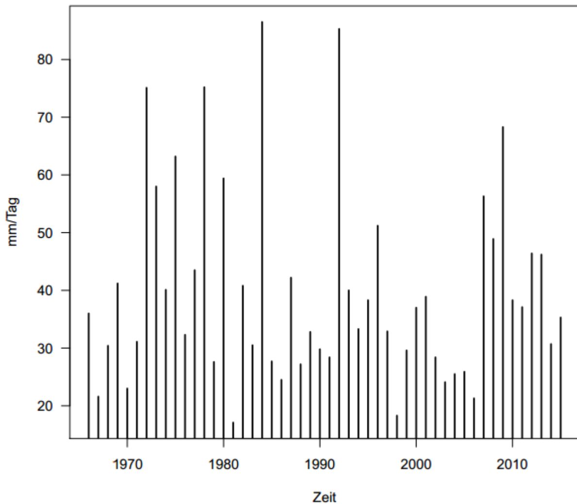
Bild 26 CH Schaffhausen, 1-Tages-Niederschlag 1966 – 2015
