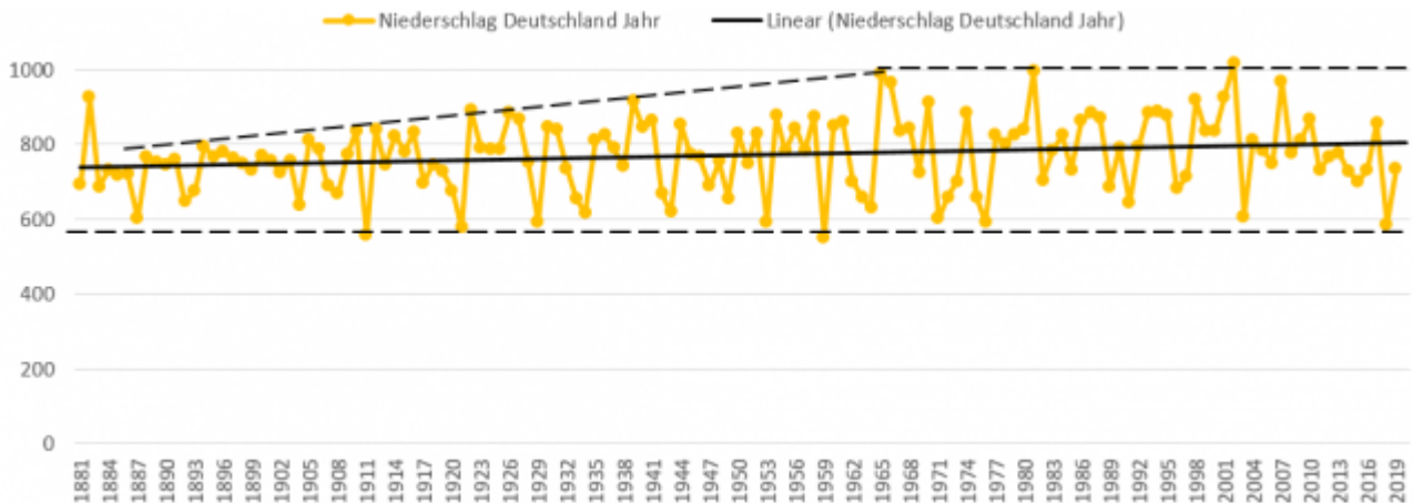
Bild 14 Deutschland, Jahresniederschlag 1881 – 2019. Grafik vom Autor erzeugt. Datenquelle: DWD Klimaviewer
