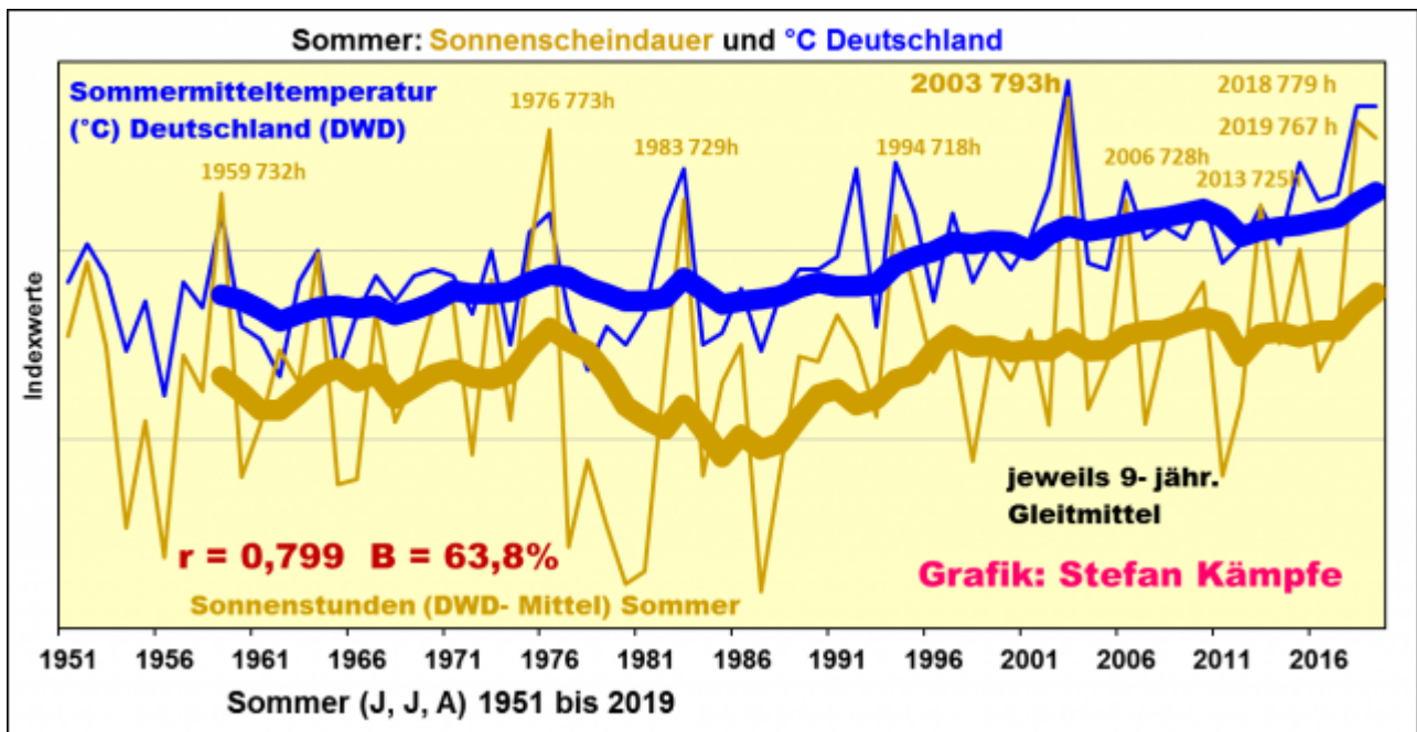
Abbildung 3: Entwicklung der Sonnenscheindauer und der Lufttemperaturen im Deutschen Flächenmittel; Daten der Sonnenscheindauer sind hierfür seit 1951 verfügbar. Umrechnung beider Messgrößen in Indexwerte.
