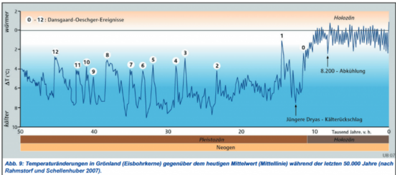
Abbildung 5: Jähe Temperatursprünge (Anstiege) um 3 bis 5 Grad in nur Jahrzehnten mit anschließender Wiederabkühlung. Bildquelle
