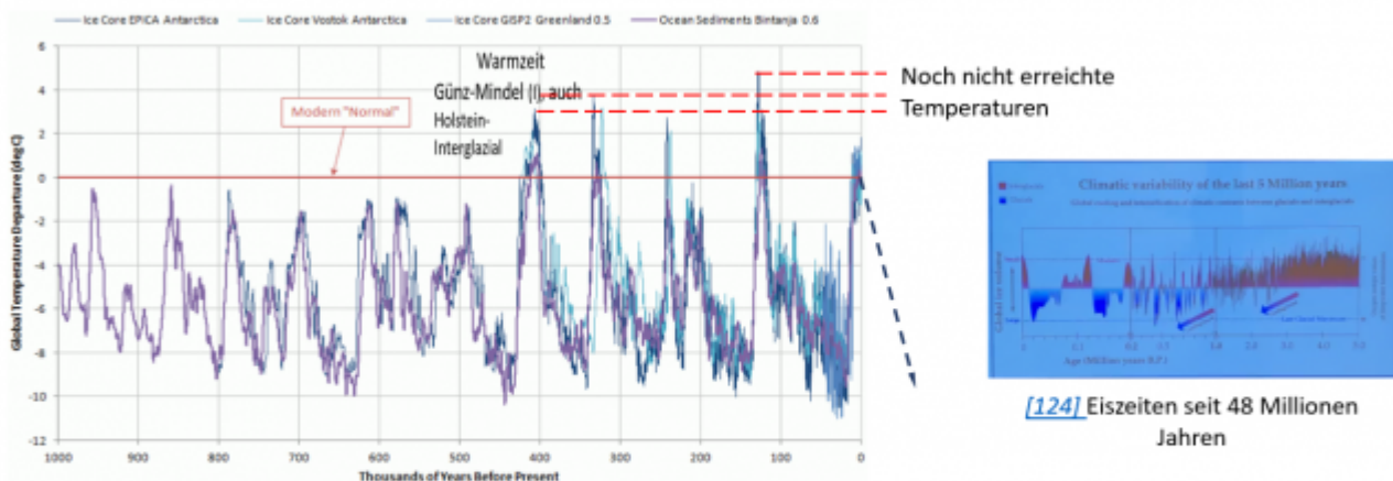
Bild: Eiszeiten der letzten 1 Millionen Jahre.
