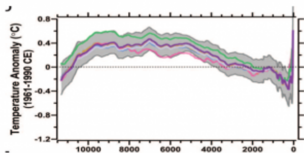
Die „gleiche“ Temperaturrekonstruktion anhand der gleichen Daten von Marcott, nun dargestellt in seiner Studie 2013
