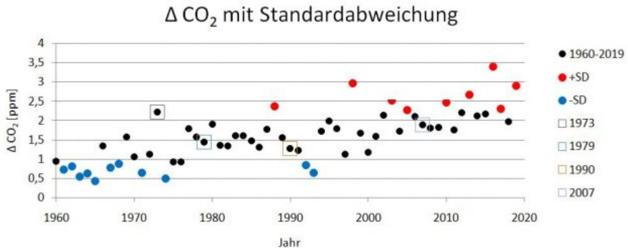
Abb. 5: Änderungen der CO 2 Konzentration zum Vorjahr. Mit der Standardabweichung sollen extreme Änderungen erkannt werden.
