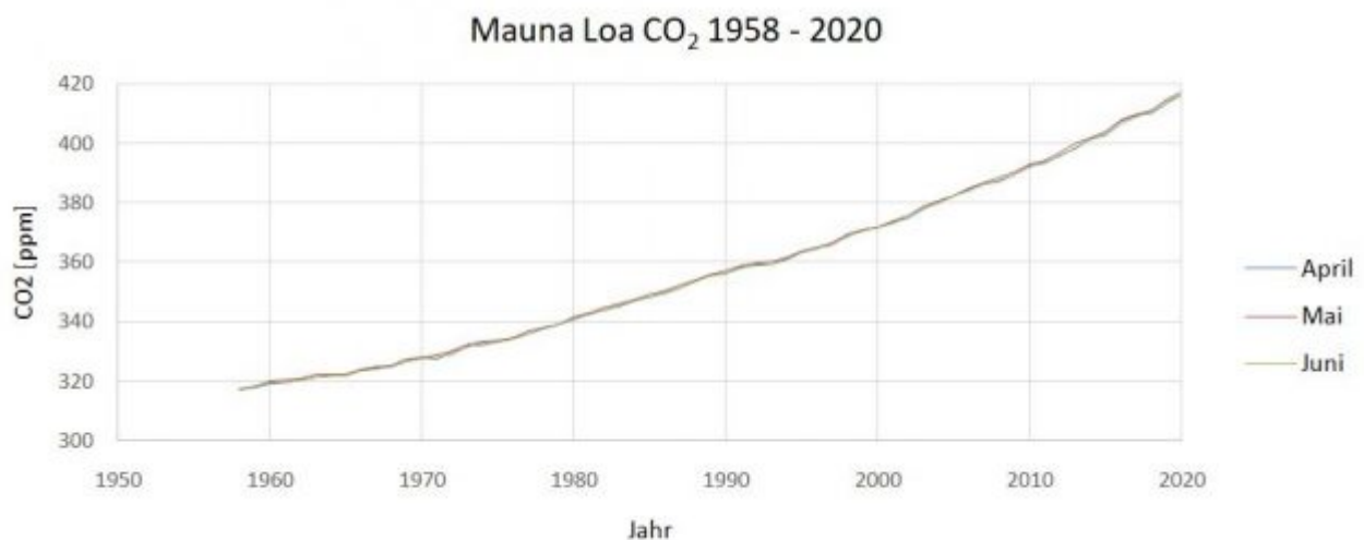
Abb. 1: Mauna Loa CO 2 1958 – 2020. Die CO 2 Konzentration ist im Beobachtungszeitraum von 317 ppm auf 417 ppm gestiegen. Also um 100 ppm in 63 Jahren. Durchschnittlich erhöhte sich die CO 2 Konzentration um 1,6 ppm/Jahr.
