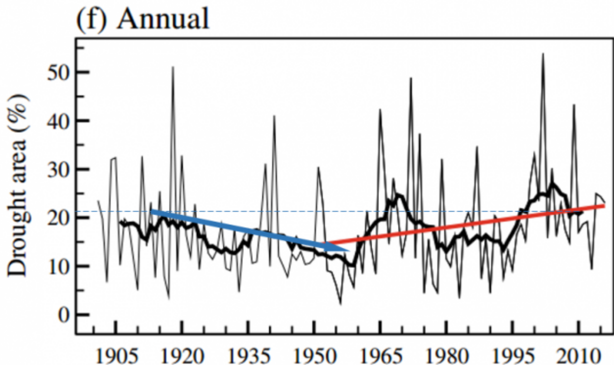
Bild 41 [11] Fig. 6.1 Indien, von Dürre betroffene Flächenanteile seit 1900 (Teilbild). Blaue Hilfslinien vom Autor zugefügt
