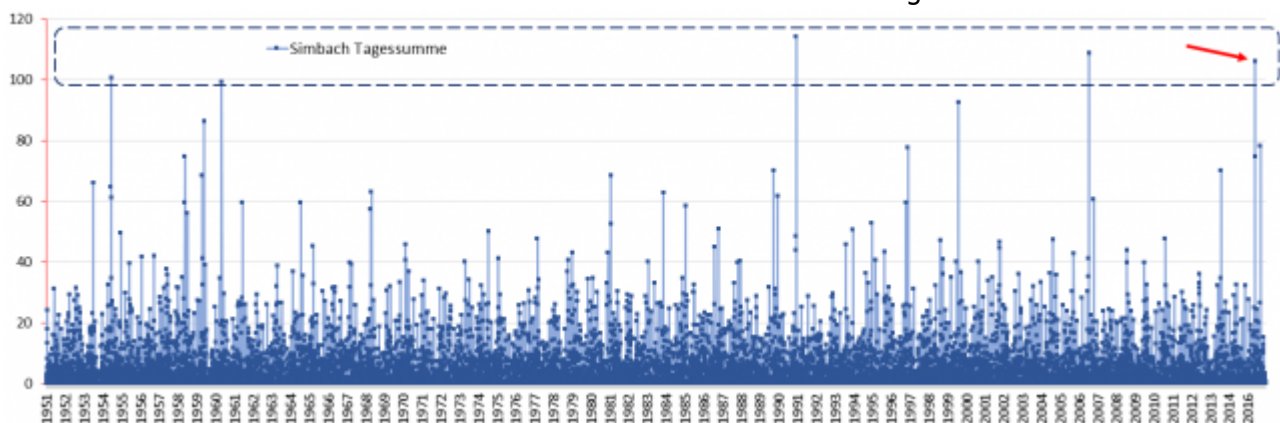
Bild 21 Simbach: Tagesverlauf Niederschlag. Der Pfeil kennzeichnet das Starkregenereignis von 2016. Grafik vom Autor anhand der DWD-Daten erstellt [4]
