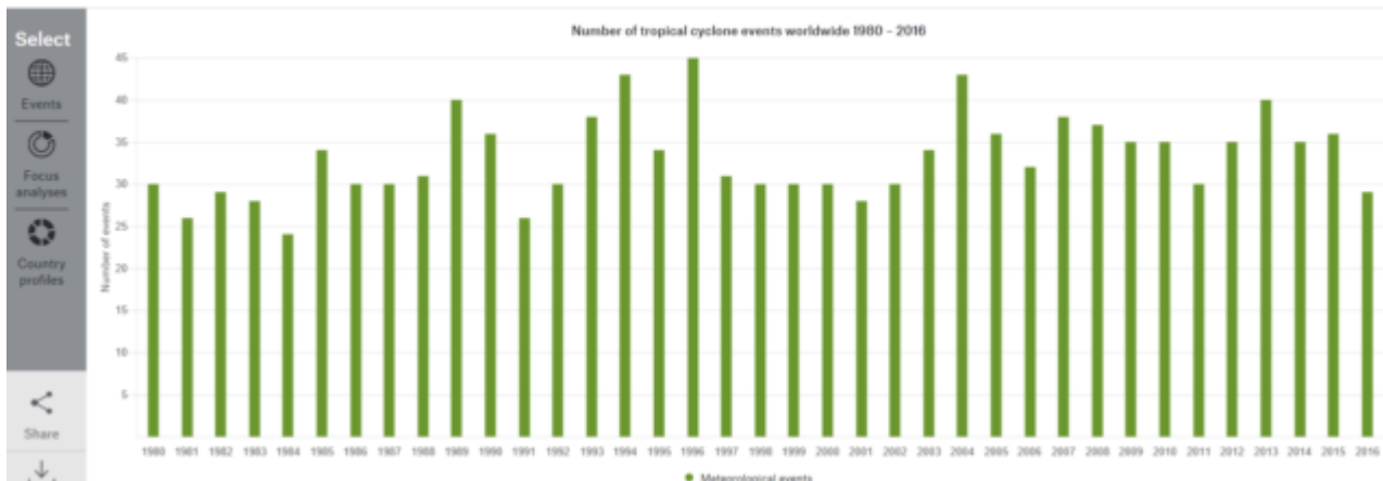
Bild 4 Anzahl tropischer Zyklone weltweit: Quelle Munich Re
