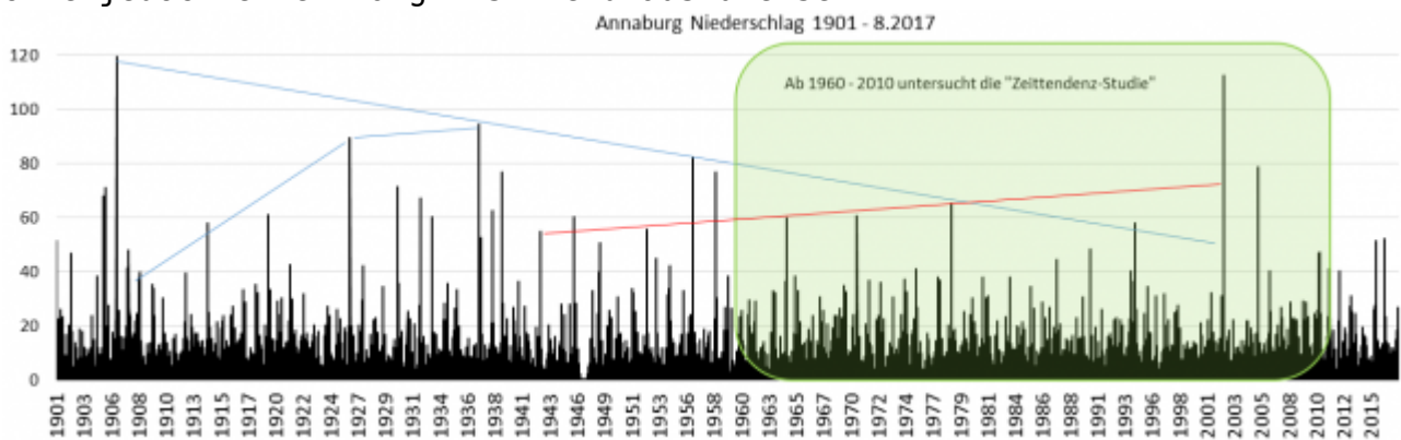
Bild 13 Tagesniederschlag Annaburg (DWD-Station 170) von 1901 – 2017
