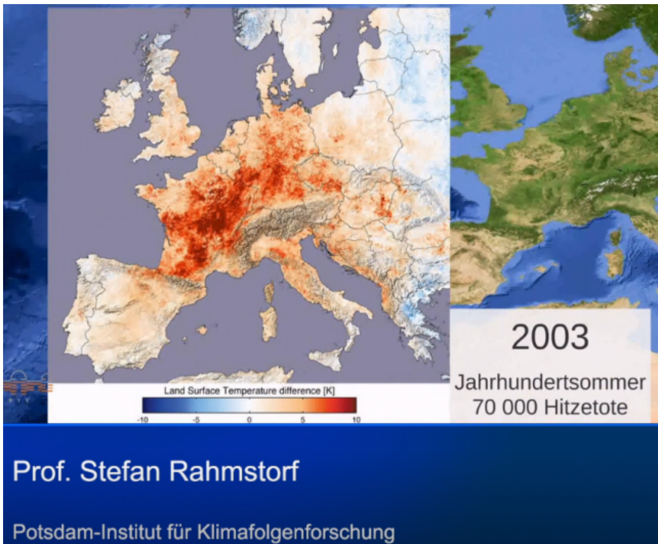
Bild 29 Bild Foliensatz Rahmstorf
