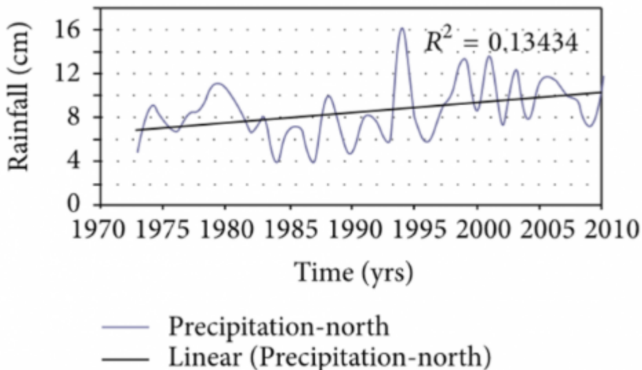
Bild 6 Niederschlagsverlauf im Norden des Sahel seit 1970 (Teilbild)
