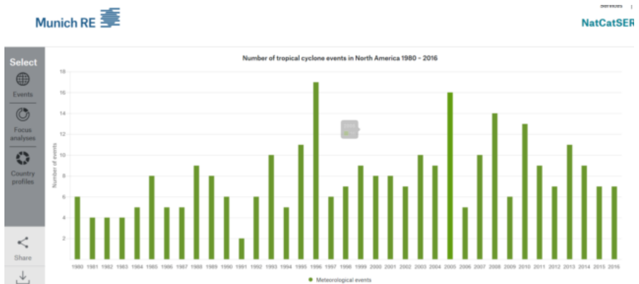
Bild 3 Anzahl tropischer Zyklone in Nord-Amerika: Quelle Munich Re
