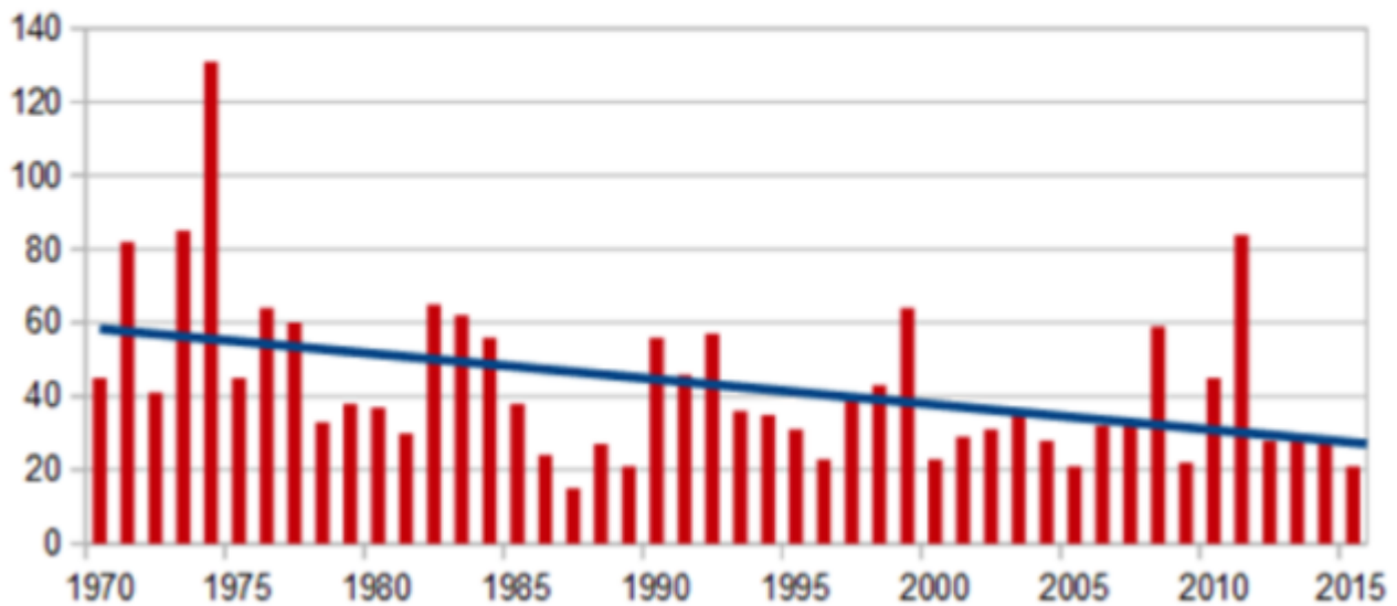
Bild 2 USA: Jährliche Tornadozahl EF-3 und stärker seit 1970
