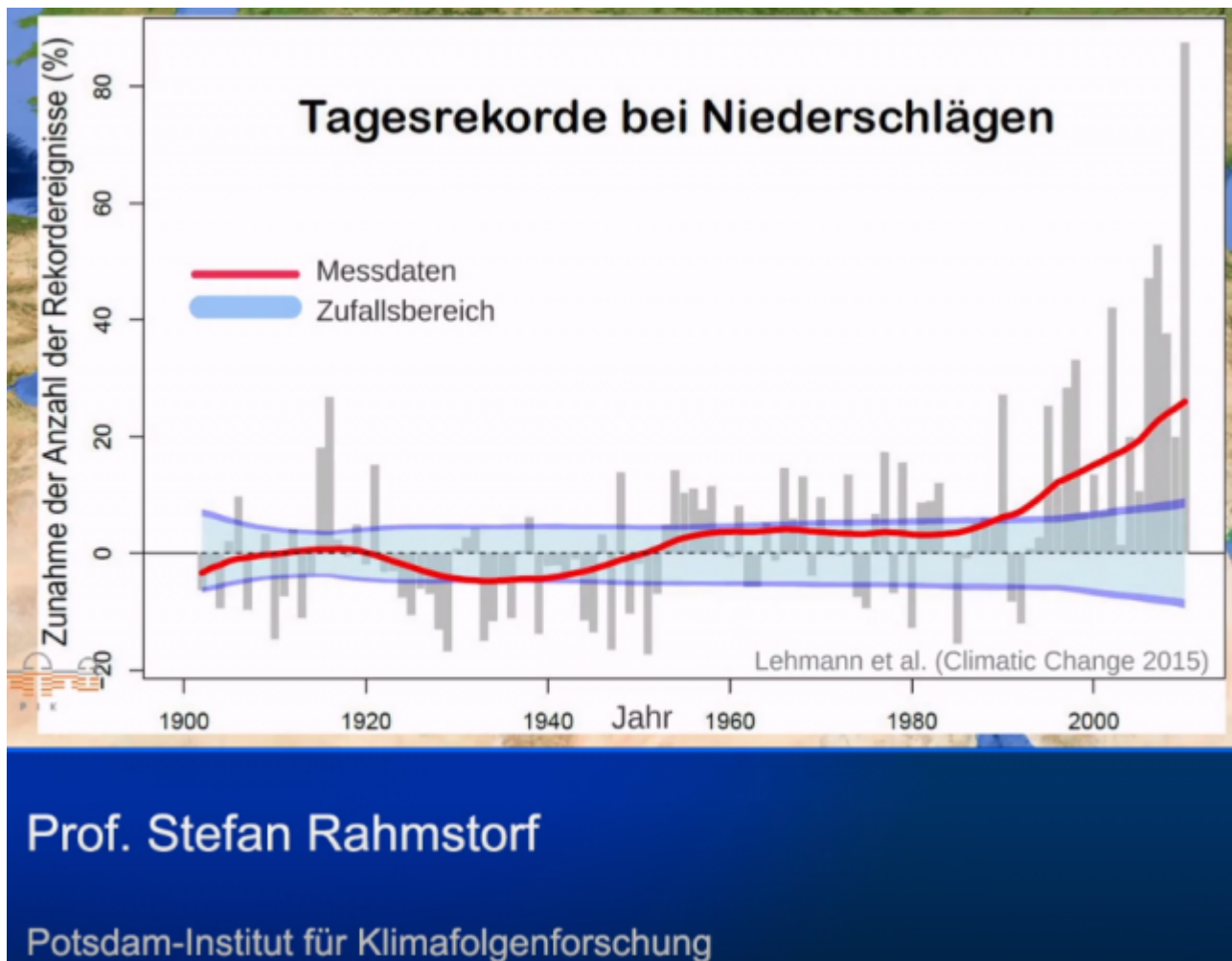
Bild 12 Extremniederschlag im Vortrag von Prof. Rahmstorf
