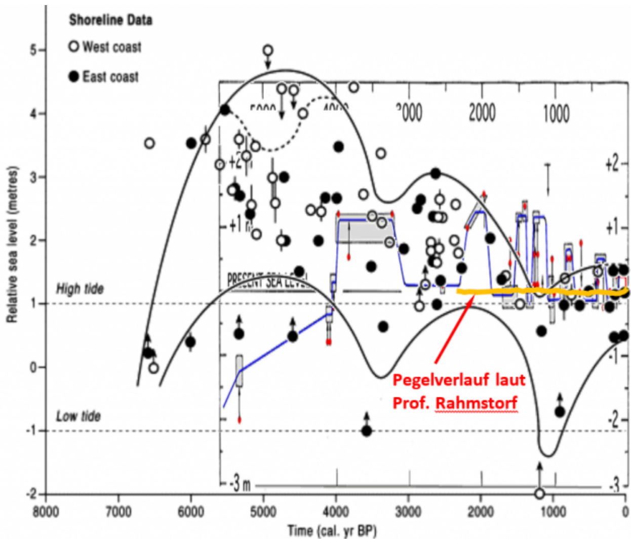
Bild 24 [5] Rekonstruktionsversuch Pegelverlauf der letzten 3000 Jahre. Bilder ([5] 3; 7; 21 im gleichen Zeit- und Höhenmaßstab vom Autor übereinander kopiert). Hinweis: Die 0-Linien der Proxi-Y-Achsen sind versetzt. Die Pegelspannen aber im Maßstab
