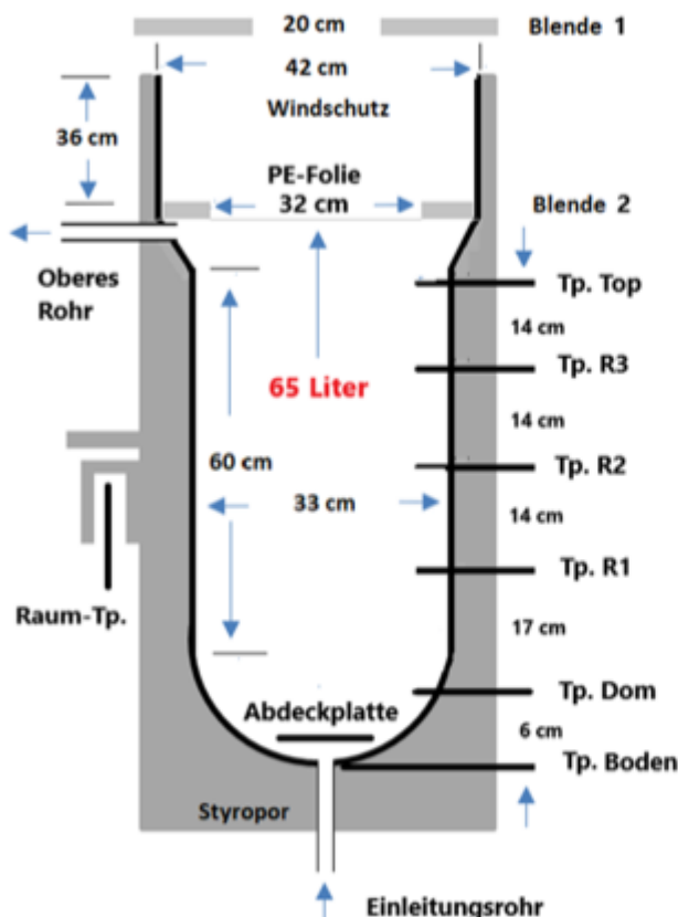
Abb. 1: Schema der Versuchsanordnung
