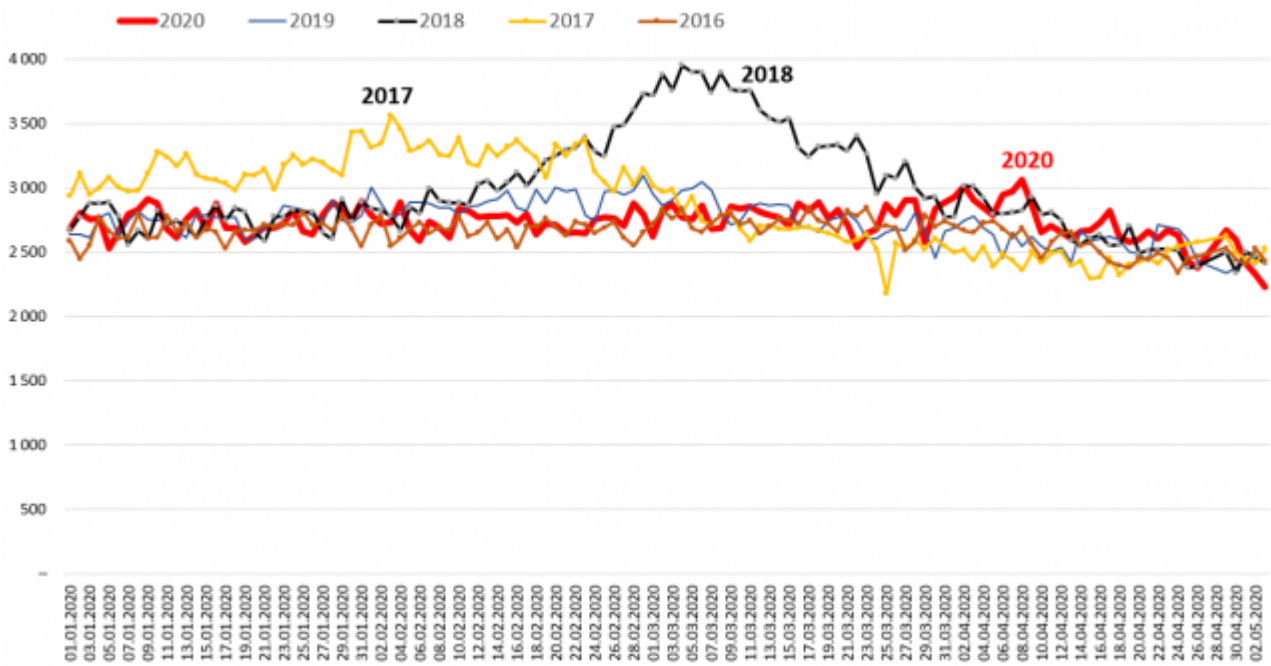
Bild 10 Grafik der Sterbedaten in Tagesauflösung mit allen Einzeljahren (um die Bevölkerungszahlen der Einzeljahre korrigiert*). Grafik vom Autor erstellt. Datenquelle: Statistisches Bundesamt, Informationsdatum 29.05.2020
