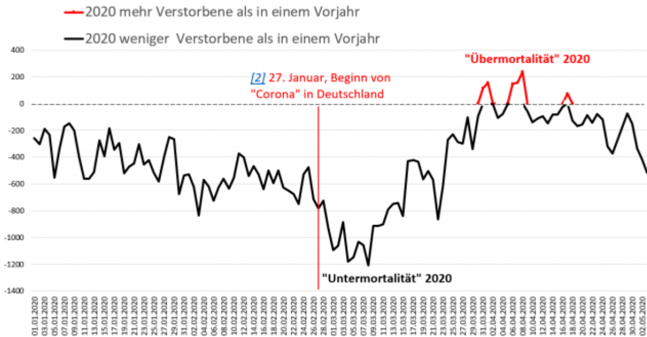
Bild 4 Grafik der Sterbedaten-Differenzen in Tagesauflösung (um die Bevölkerungszahlen der Einzeljahre korrigiert*). Grafik vom Autor erstellt. Datenquelle: Statistisches Bundesamt, Informationsdatum 29.05.2020
