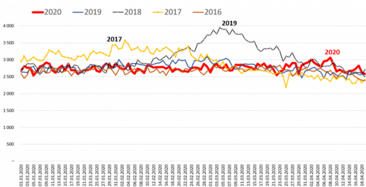
Bild 7 Grafik der Sterbedaten in Tagesauflösung mit allen Einzeljahren (um die Bevölkerungszahlen der Einzeljahre korrigiert*). Grafik vom Autor erstellt. Datenquelle: Statistisches Bundesamt, Informationsdatum 15.05.2020
