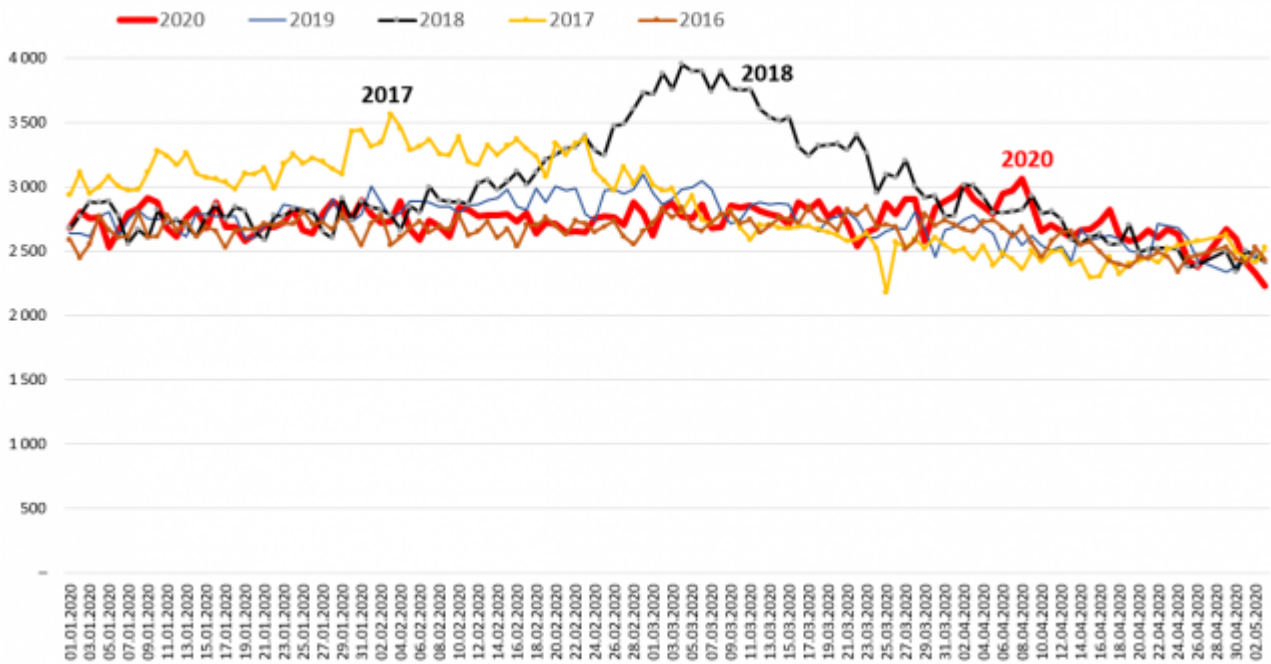
Bild 2 Grafik der Sterbedaten in Tagesauflösung mit allen Einzeljahren (um die Bevölkerungszahlen der Einzeljahre korrigiert*). Grafik vom Autor erstellt. Datenquelle: Statistisches Bundesamt, Informationsdatum 29.05.2020
