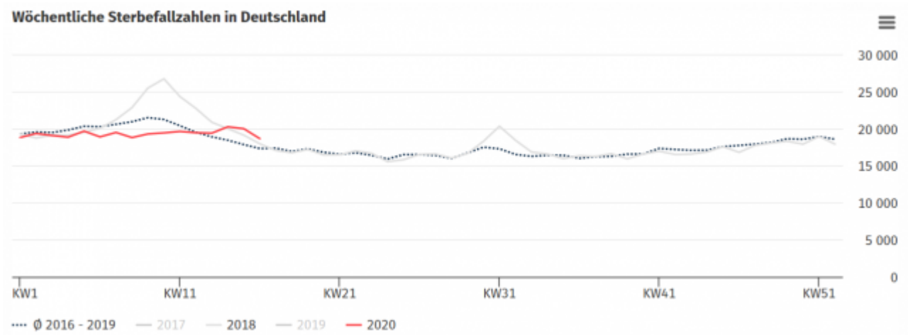
Bild 6 Grafik der Sterbedaten in Wochenauflösung. Bildquelle Statistisches Bundesamt, Informationsdatum 15.05.2020
