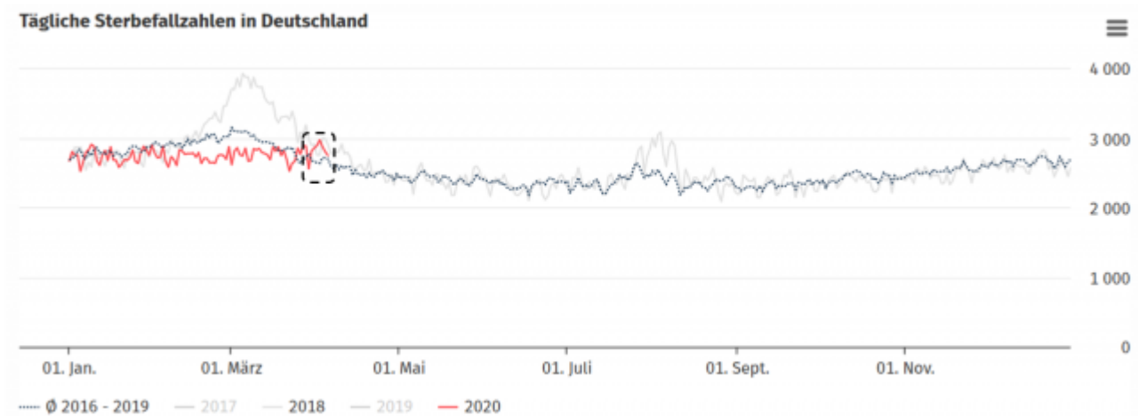
Bild 5 [1] Grafik der Sterbedaten des Statistischen Bundesamtes der letzten Märzwoche. Schwarze Umhüllung des Zeitraumes „seit der letzten Märzwoche“ vom Autor zugefügt
