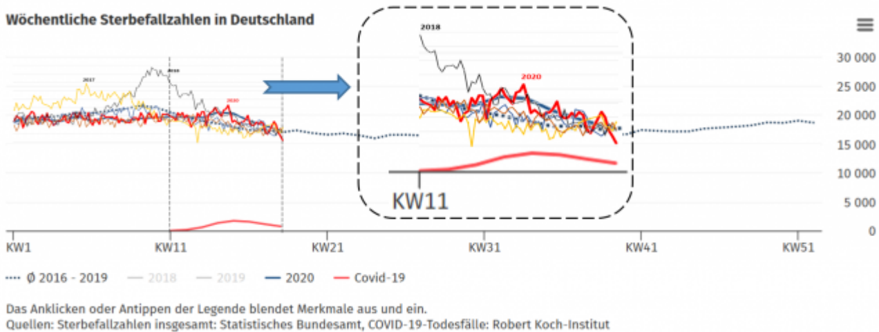
Bild 3 Bilder 2 und 3 übereinander kopiert. Bereich der Corona-„Übermortalität“ zusätzlich gezoomt dargestellt. Grafik vom Autor erstellt
