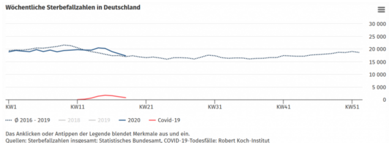
Bild 1 Grafik der Sterbedaten. Quelle Statistisches Bundesamt, Informationsdatum 29.05.2020
