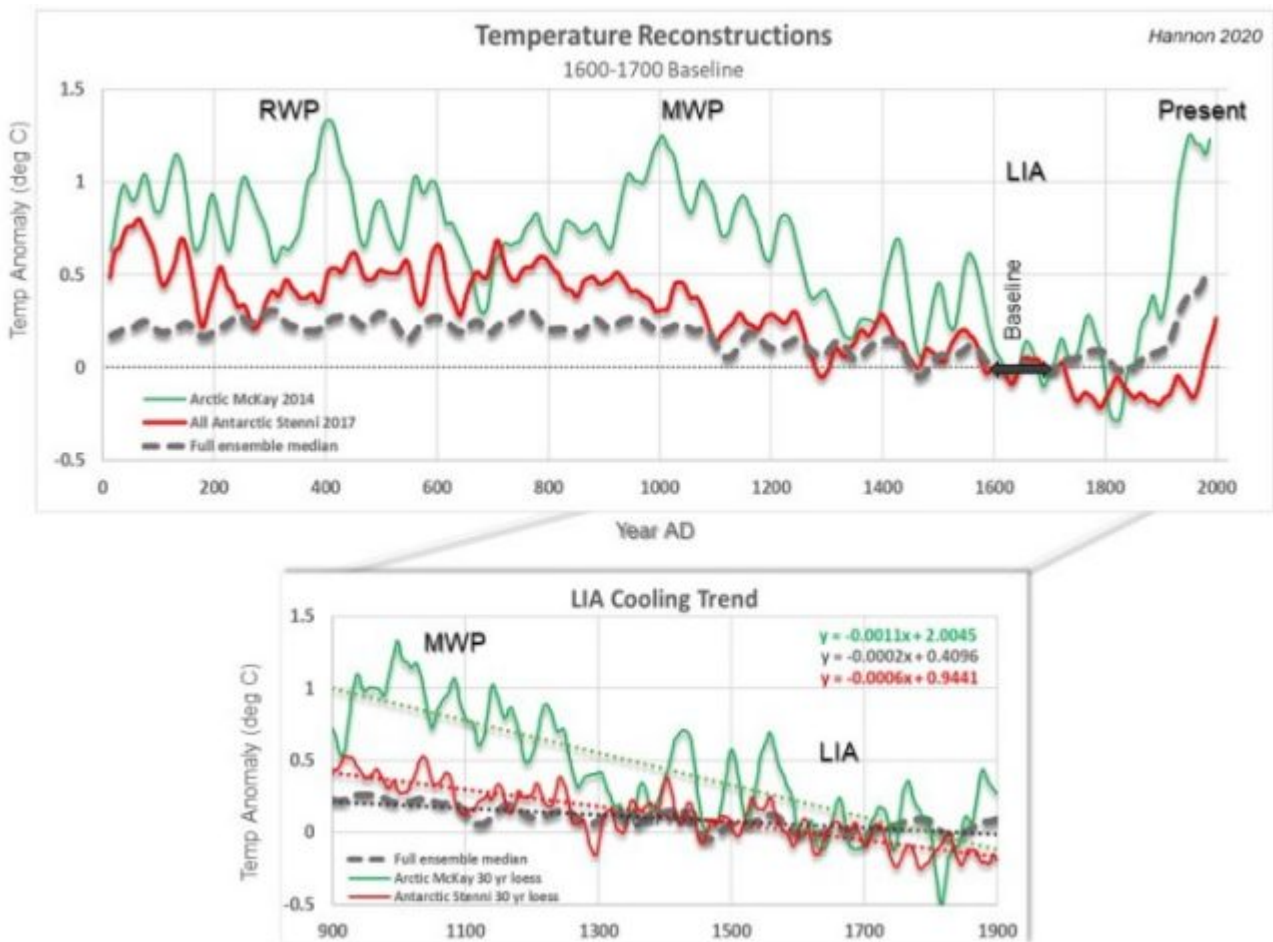
Abbildung 2: Temperatur-Rekonstruktionen von Arktis und Antarktis der globalen Mittelwerte nach Pages 2K im Vergleich zum Referenzzeitraum 1600 bis 1700. Die Rekonstruktionen sind mit einem 50-Jahre-Loess-Filter versehen. Die untere Graphik ist eine Vergrößerung, welche lineare Trends von der MWP zur LIA zeigt. Diese Rekonstruktionen sind mit einem 30-Jahre-Loess-Filter versehen.
