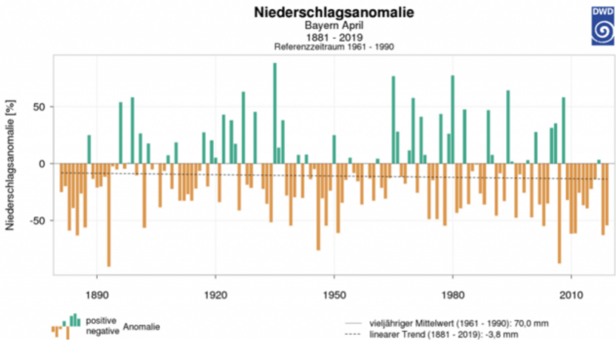
Bild 11 April-Niederschlagsanomalie Bayern seit 1881. Quelle: DWD-Viewer
