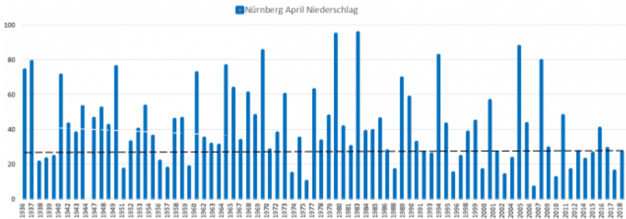
Bild 21 Nürnberg Niederschlag April ab 1936. Quelle: DWD-Daten. Grafik vom Autor erstellt
