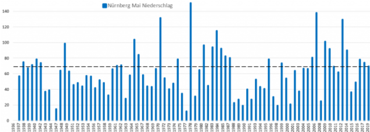
Bild 20 Nürnberg Niederschlag Mai ab 1936. Quelle: DWD-Daten. Grafik vom Autor erstellt
