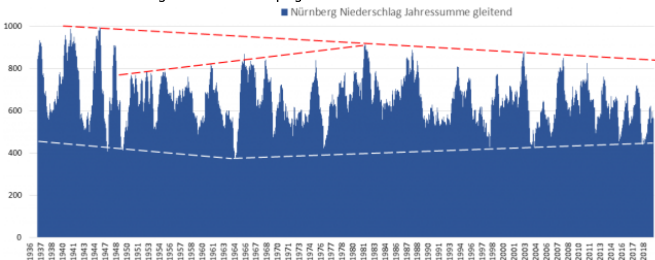
Bild 15 Nürnberg Niederschlag Jahressumme gleitend ab 1936. Quelle: DWD-Daten. Grafik vom Autor erstellt
