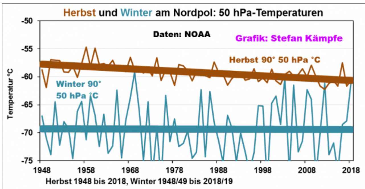
Abbildung 3: Merklicher Rückgang der 50 hPa-Stratosphärentemperatur am Nordpol seit 1948 (keine längere Datenverfügbarkeit) im Herbst; fast kein Trend im Winter. Aber im Winter kann die nachlassende Sonnenaktivität auch keinen direkten Einfluss mehr haben, da die Sonne dann nicht scheint (Erdschatten über dem Pol). Es ist aber denkbar, dass die im Herbst kälter werdende Stratosphäre die Westwind-Zirkulation des Winters „ankurbelt“. Man beachte außerdem, dass hier nur der nördlichste Gitterpunkt betrachtet wurde; der gesamte Polarwirbel ist viel größer und in seiner Form sehr variabel; außerdem beeinflussen auch die QBO und weitere Faktoren, wie er sich verhält.
