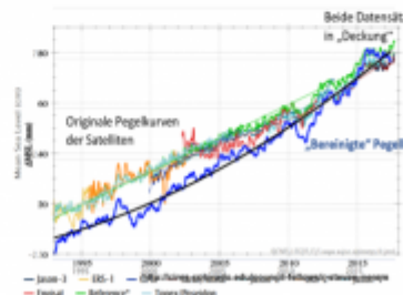
Darstellung der Satellitenpegel und eine nachträgliche „Fehlerbereinigung“ aus einer Studie [6]. Grafik vom Autor zusammengestellt
