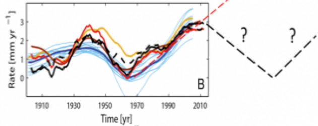
Tidenpegel-Änderungsrate Verlaufsdarstellung in einer im IPCC-Bericht als Beleg gelisteten Studie, Dangendorf et al., 2017. Bild vom Autor ergänzt
