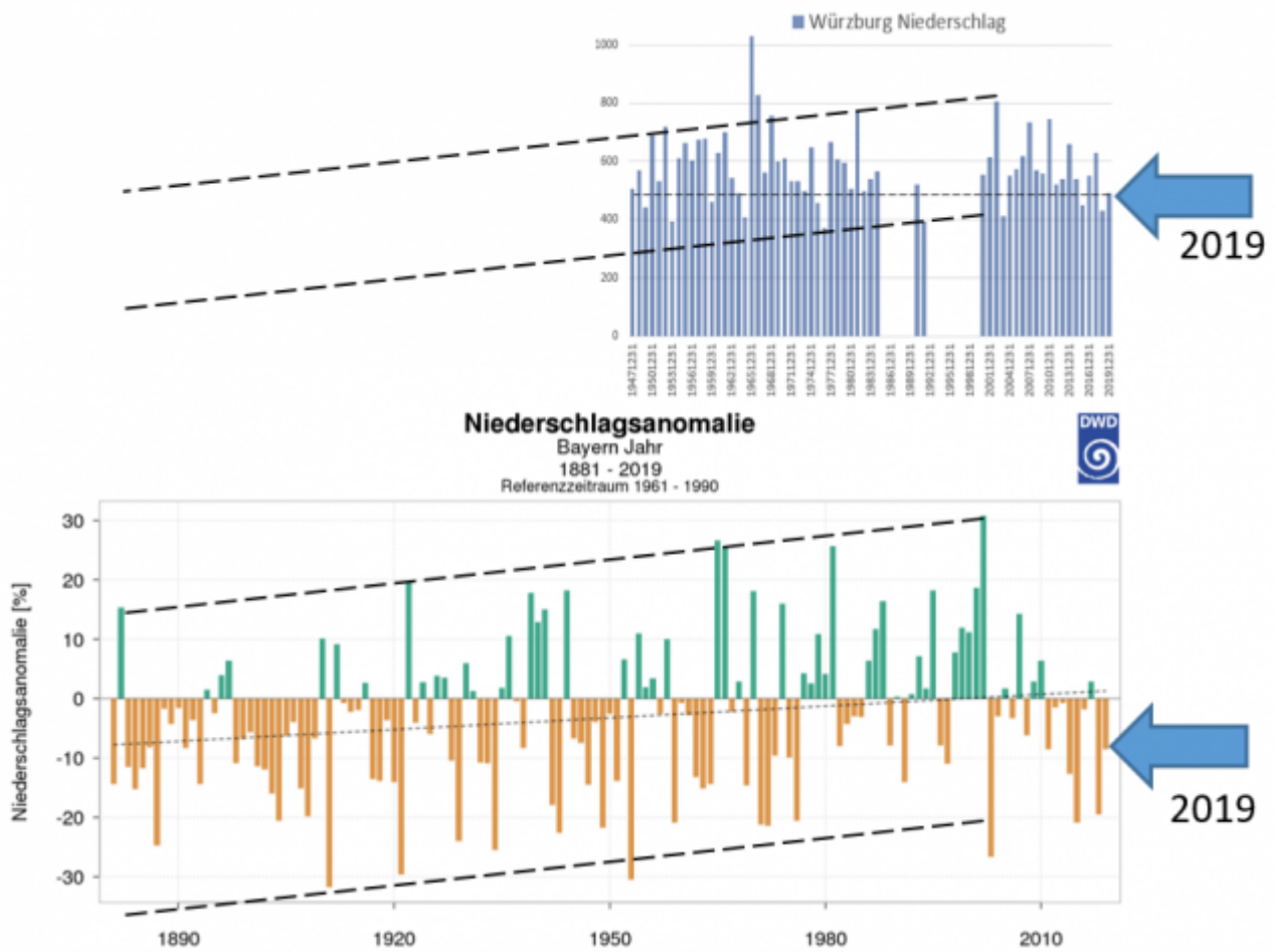
Bild 1 Jahresniederschlag Würzburg ab 1947 und Bayern ab 1881. Grafik vom Autor teils erstellt, ergänzt und zusammengefügt. Quellen: DWD
