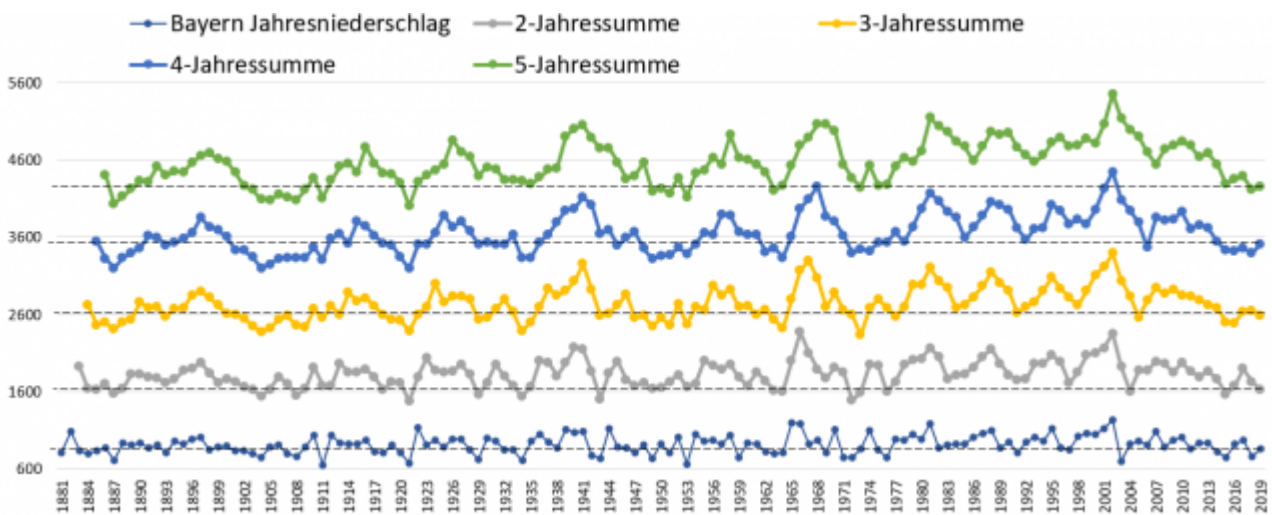
Bild 6 Bayern, mehr-Jahresniederschläge seit 1881. Grafik vom Autor anhand der DWD-Daten erstellt
