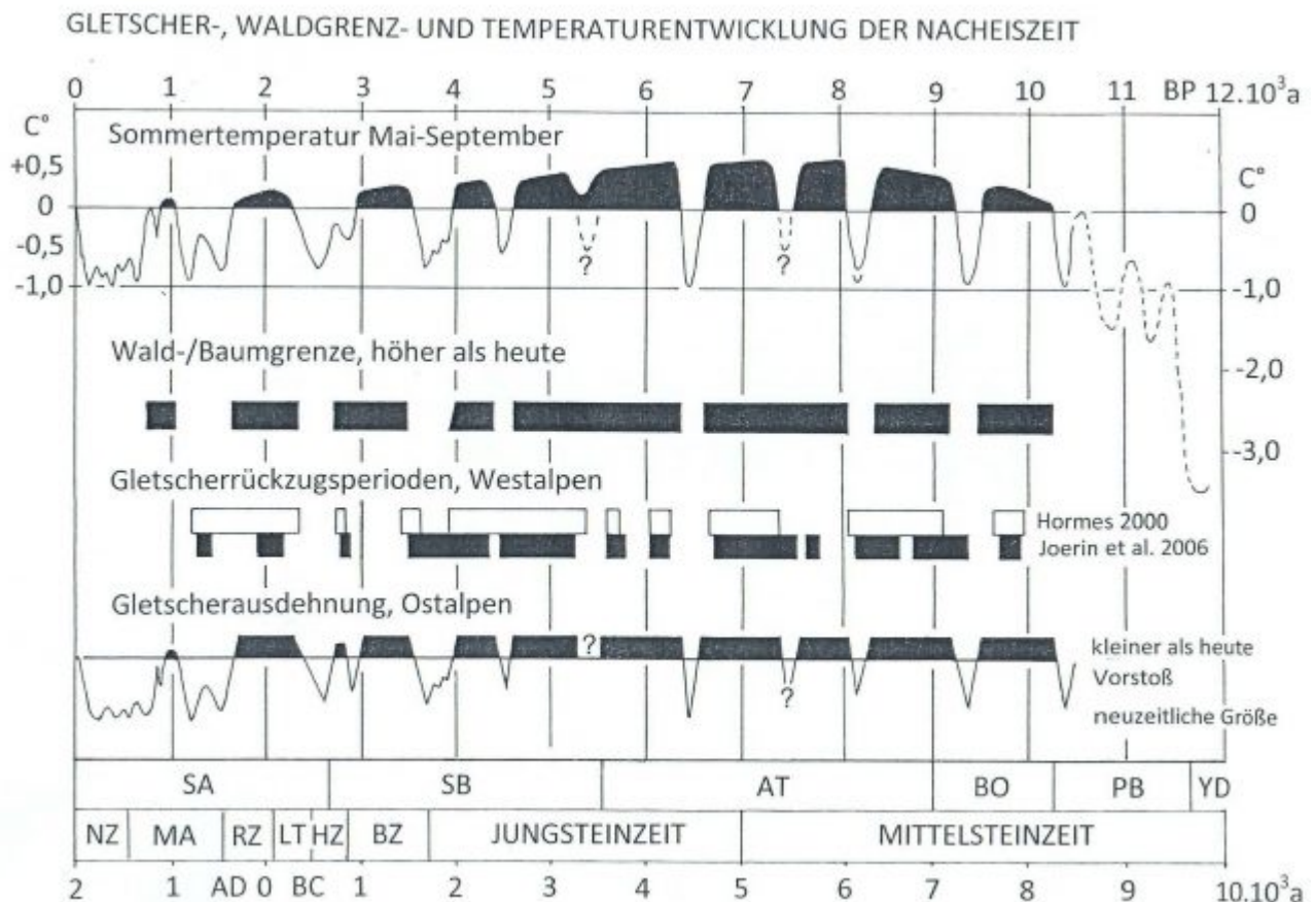
Bild 1: Sommertemperatur, Wald-/Baumgrenze, Gletscherrückzugsperioden Westalpen, Gletscherausdehnung Ostalpen, Grafik aus S. 238 des besprochenen Buchs von G. Patzelt.
