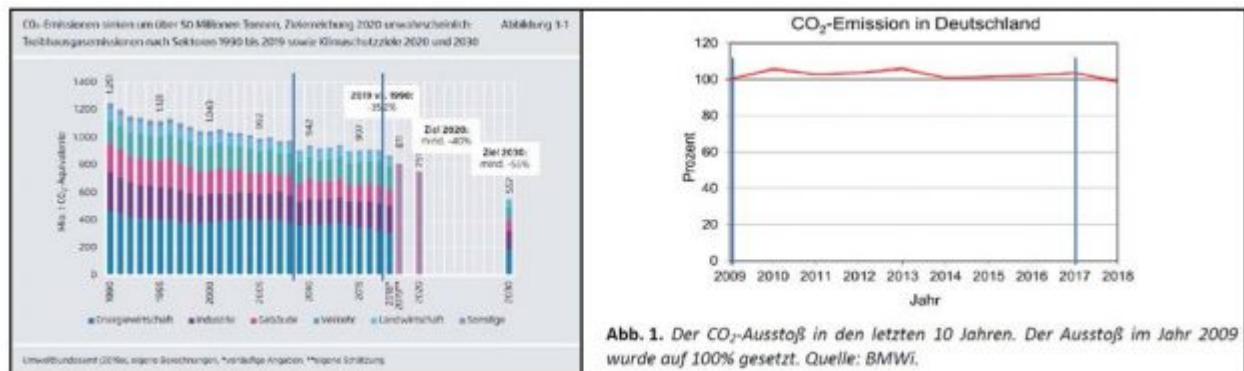
Bild 1: CO 2 -Emissionen in Deutschland. Links: AE, S. 25, Abb. 3-1. Rechts: Uni-HD, Abb. 1. Die senkrechten blauen Striche bei den Jahren 2009 und 2017 wurden von der Verfasserin eingezeichnet, um den Zeitraum in drei Phasen zu gliedern und den visuellen Vergleich der Grafiken zu erleichtern.
