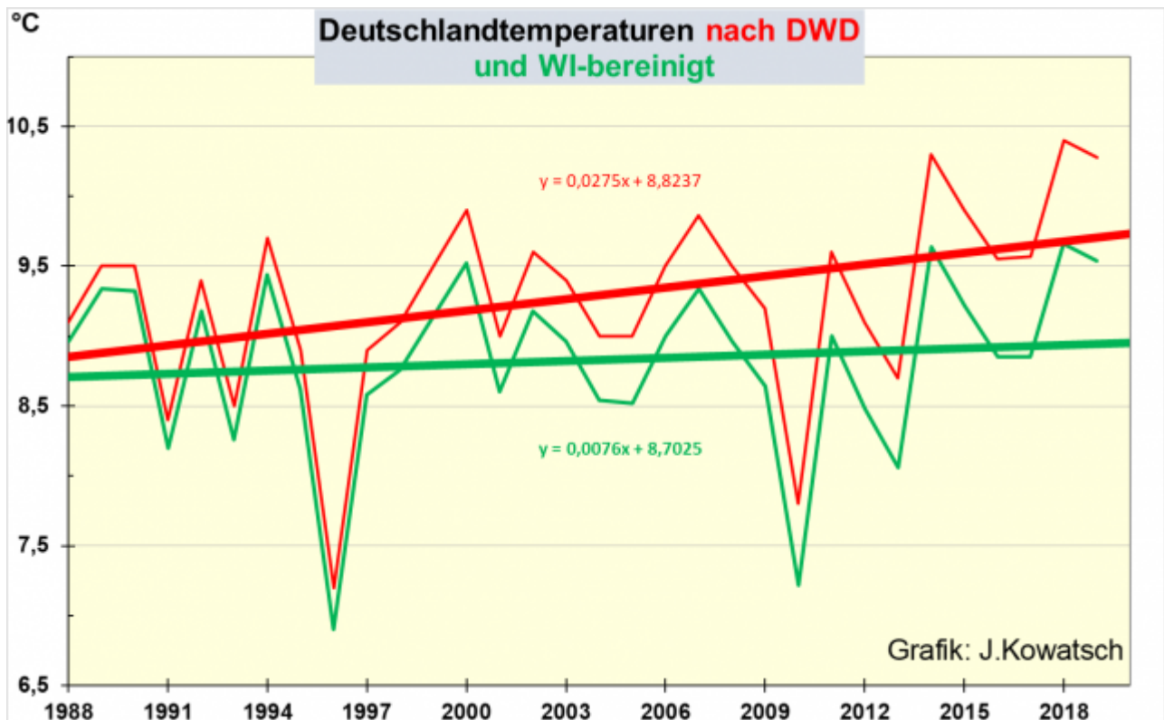
Abb. 5: Die grüne Temperaturkurve ist wärmeinselbereinigt. So könnte der
