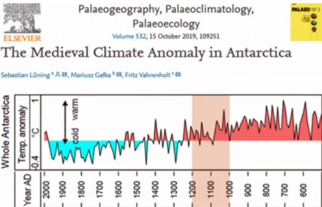
Bild 42 Quelle: NoTricksZone
