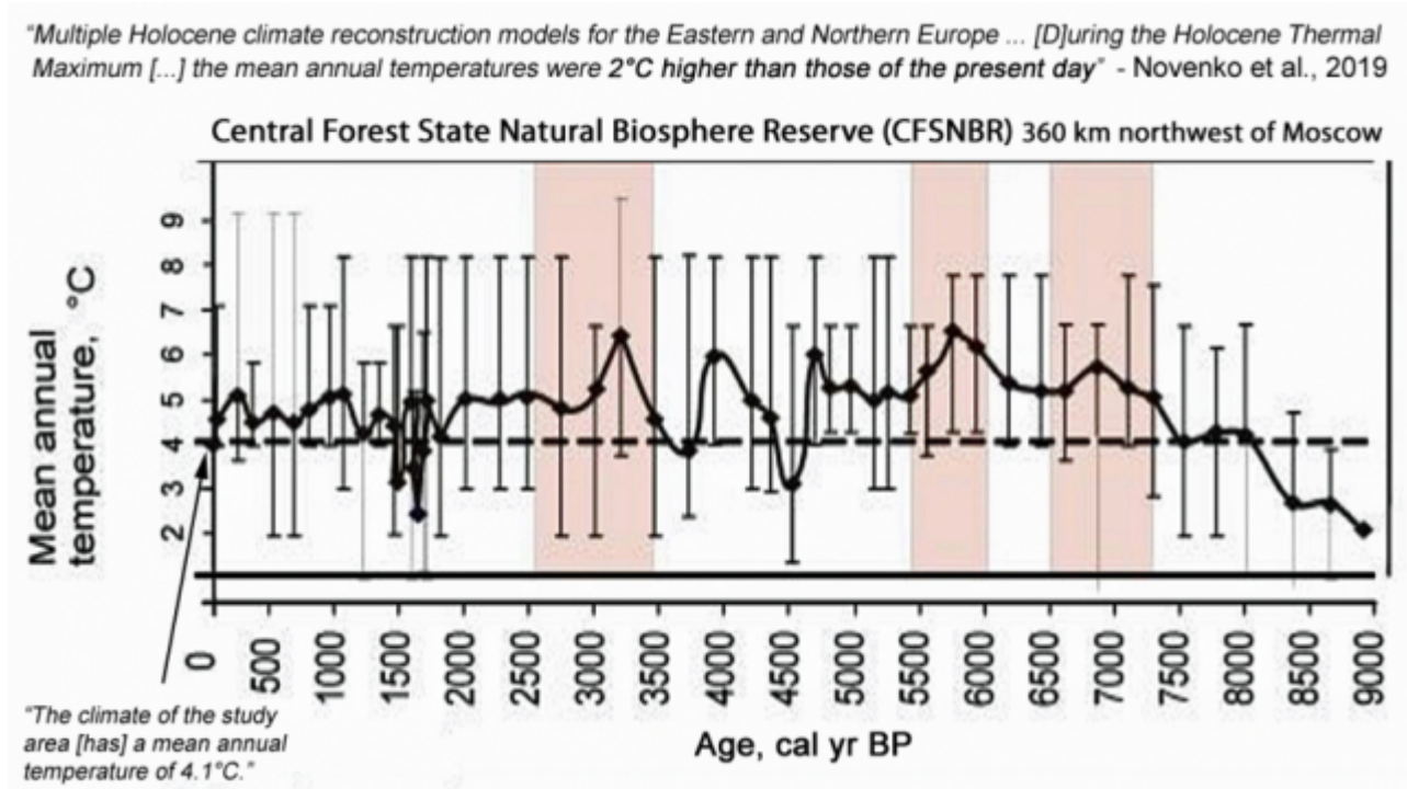
Bild 40 Quelle: NoTricksZone
