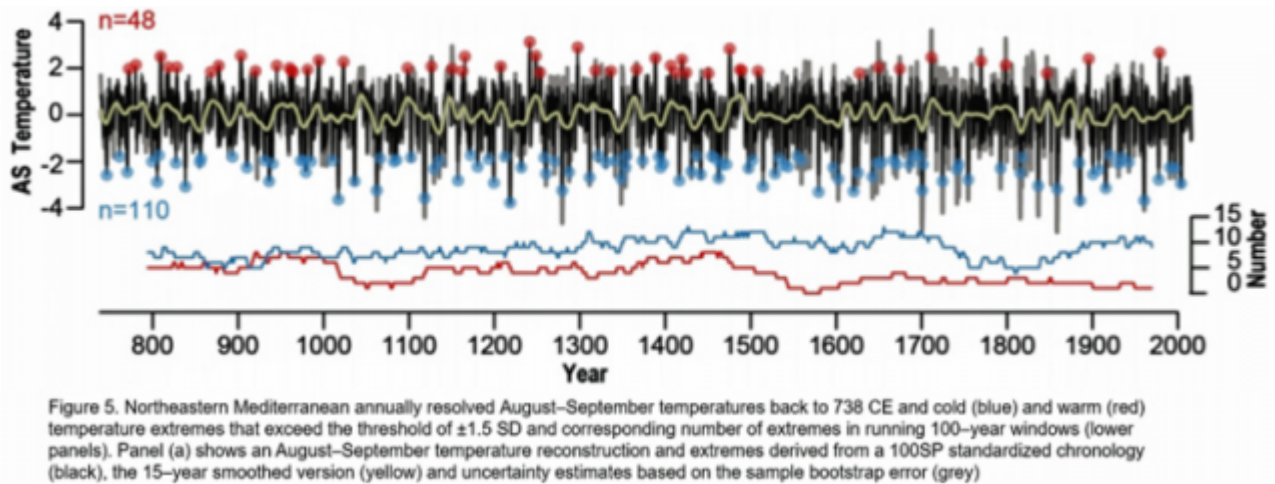
Bild 36 Quelle: NoTricksZone
