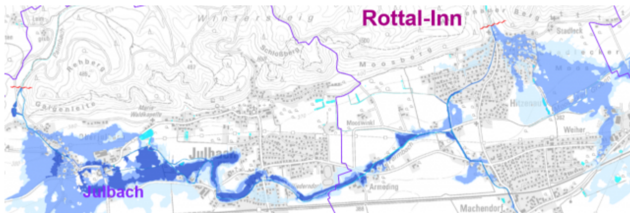
Bild 16 Flurbild mit eingezeichneten Hochwassergefahrenflächen bei
