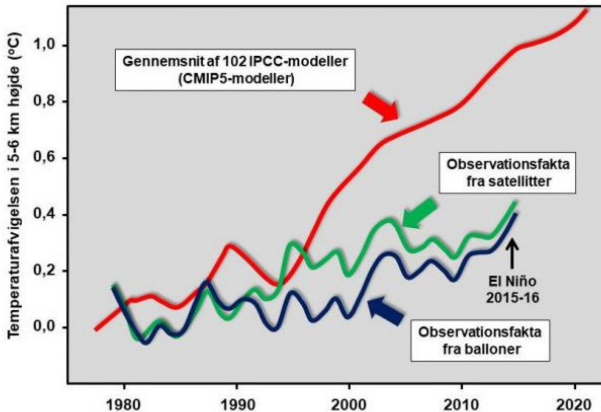
Abbildung 3. Vergleich zwischen Beobachtungen von Ballonen und Satelliten und dem Durchschnitt der Temperaturabweichung von 102 Klimamodellen ab 1979 bei 5–6 km über den Tropen für den Zeitraum 1979–2016. Die Grafik wurde von Atmosphärenforscher John Christy während einer Anhörung im US-Repräsentantenhaus präsentiert. Quelle: J. R. Christy 2017: Annahmen, politische Implikationen und die wissenschaftliche Methode. Climate Science .
