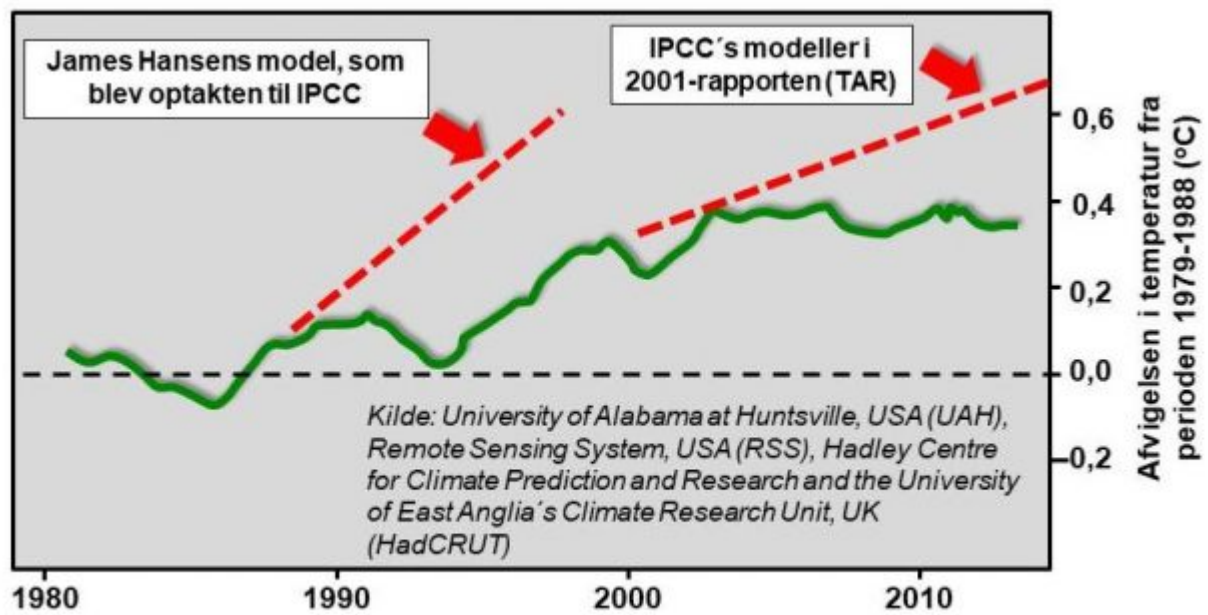
Abbildung 2. Sowohl das Modell von James Hansen als auch das Modell im 3. IPCC-Bericht aus dem Jahr 2001 weichen von den Beobachtungen ab, die durch die grüne Kurve dargestellt werden. Sie zeigt den Trend der globalen Jahrestemperatur 1980–2014 als gleitender Durchschnitt der monatlichen Durchschnittswerte aus den drei am häufigsten verwendeten Datensätzen. Bis etwa 2002 steigt die Temperatur allmählich an, danach hört der globale Temperaturanstieg auf. Quelle: University of Alabama in Huntsville, USA (UAH), Fernerkundungssystem, USA (RSS) und Hadley Center für Klimavorhersagen und -forschung an der Climate Research Unit der University of East Anglia, Großbritannien (HadCRUT).
