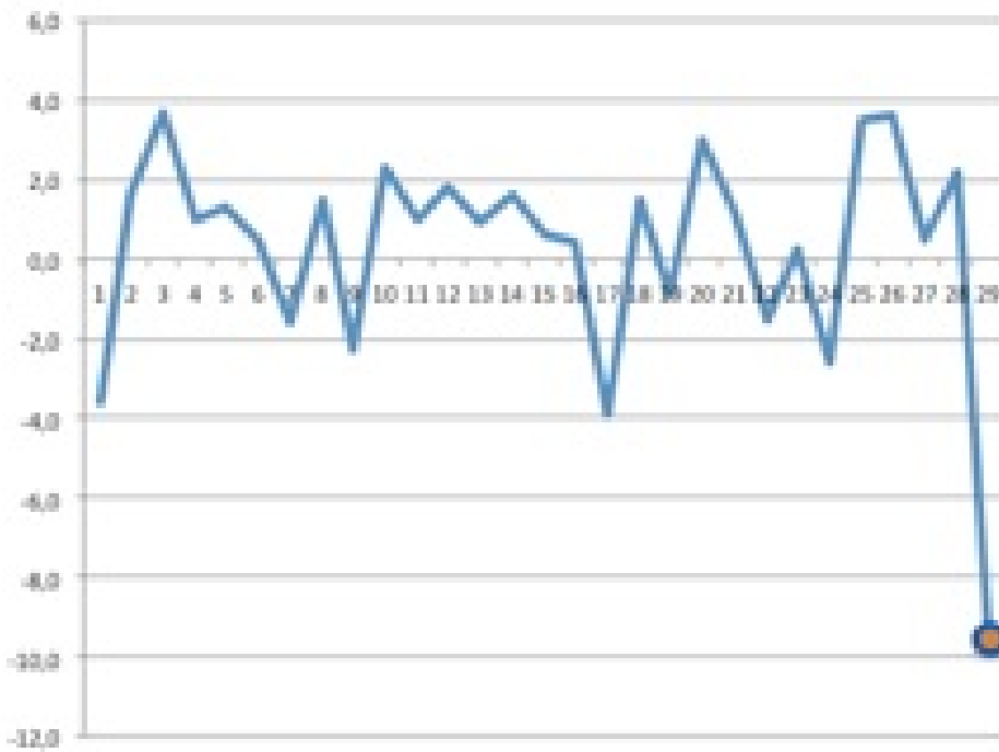
Abb. 3 Februar-Temperatur-Abweichungsmittel aus De Bilt + Berlin + Wien vom 190jährigen Mittelwert 1761-1950 ( LINKES Meteorologisches Taschenbuch ) ; Abszisse: Celsiusgrad-Einheiten; Ordinate: Zahl der Jahre nach 1900
