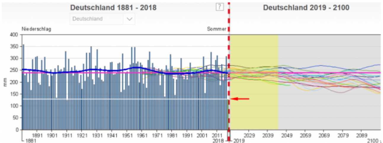
Bild 4 Sommerniederschlag Deutschland seit 1881. Der rote Pfeil kennzeichnet den Sommerniederschlag 2018. Quelle: DWD-Viewer, vom Autor ergänzt
