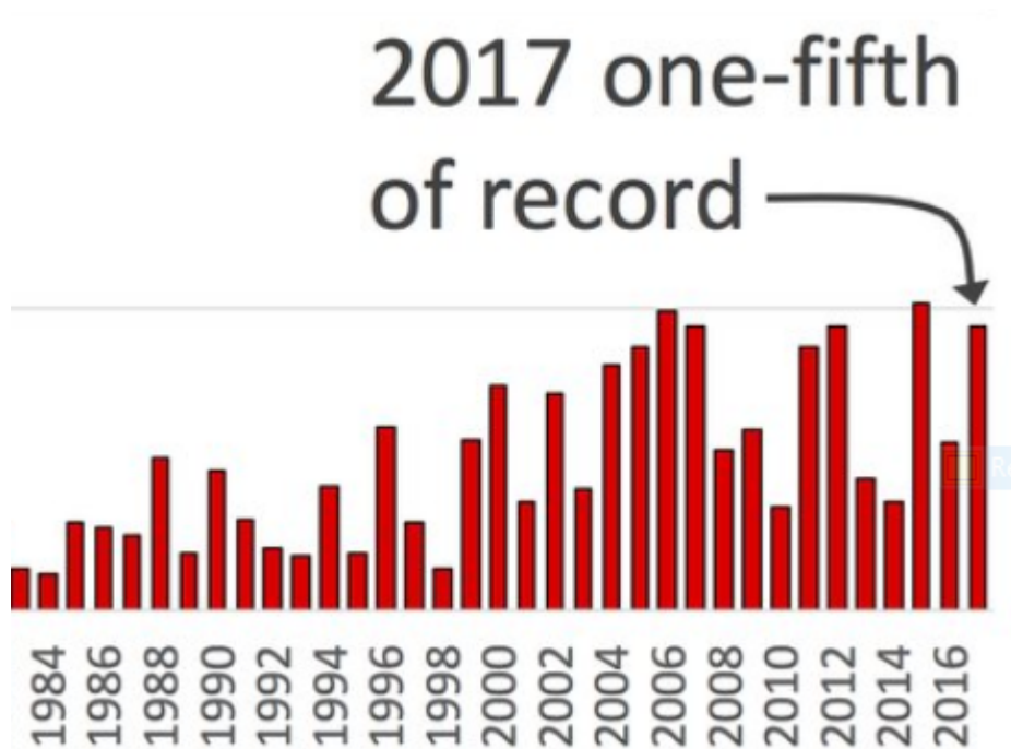
Bild 4 [4] US Wald-Brände nach Brandfläche 1984 ... 2017
