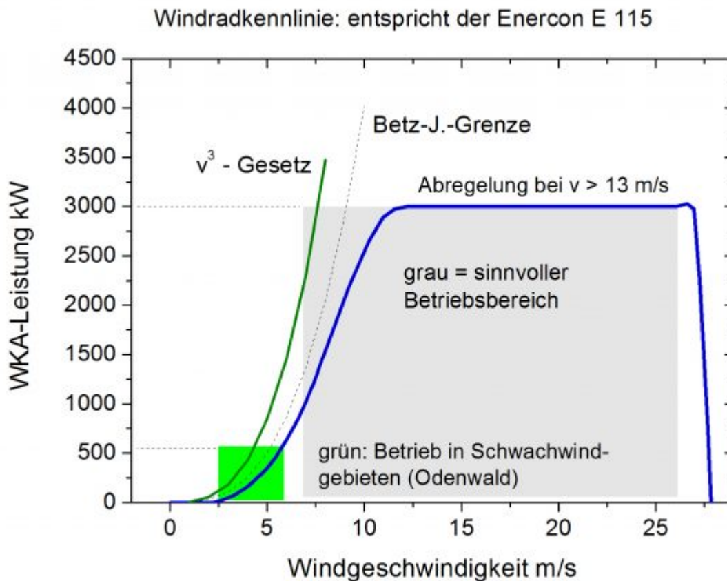
Bild 4: Beispiel einer Windradkennlinie (blau), erstellt aus den Daten [18]. Das v^3 Gesetz und die Betz-Joukowski-Grenze [32] werden prinzipiell von einem Windrad nicht erreicht. Die mittleren Windgeschwindigkeiten an der Nordseeküste [33] liegen bei 5,8 bis 5,9 m/s, für den Offshorebereich der Nordsee [34] um die 9 m/s. Selbst Offshore-Windgeschwindigkeiten lassen daher die Nutzung des sinnvollen Betriebsbereichs von Windturbinen (grau) nur eingeschränkt in dessen linken Randbereich zu.
