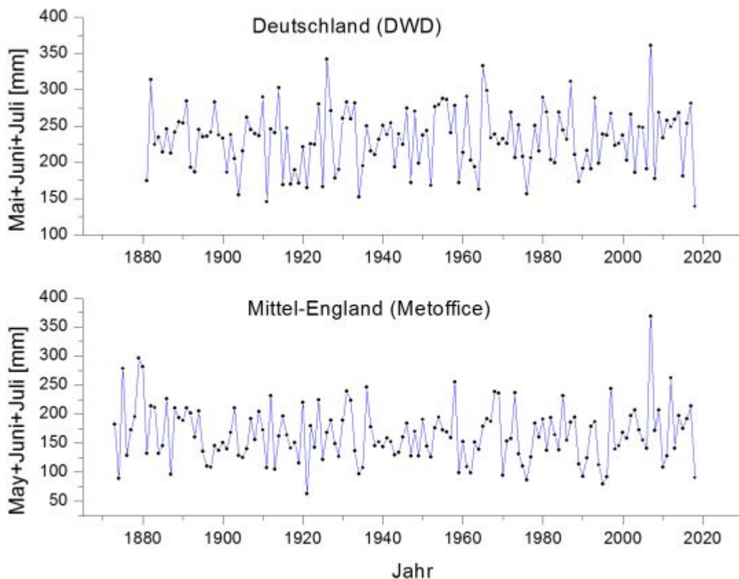
Bild: Summe der Niederschlagsmengen von Mai+Juni+Juli für Deutschland
